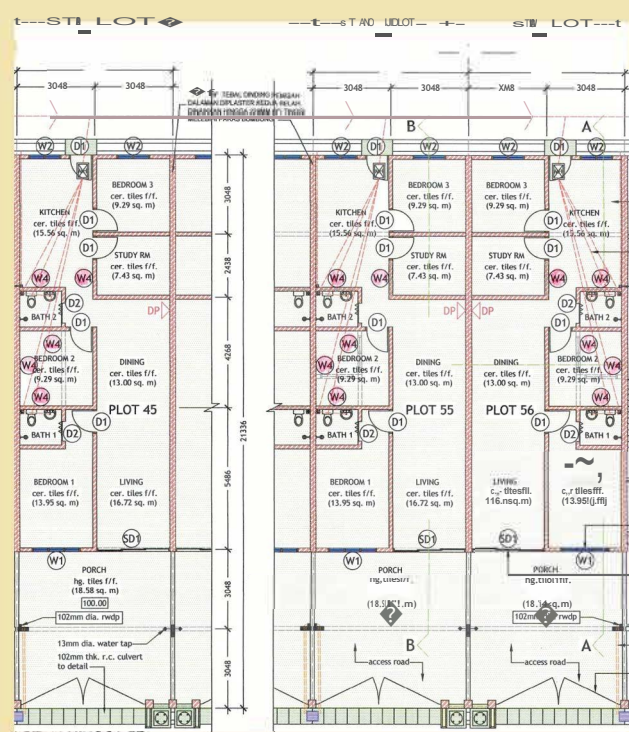
PELAN LANTAI SKALA 1:100
