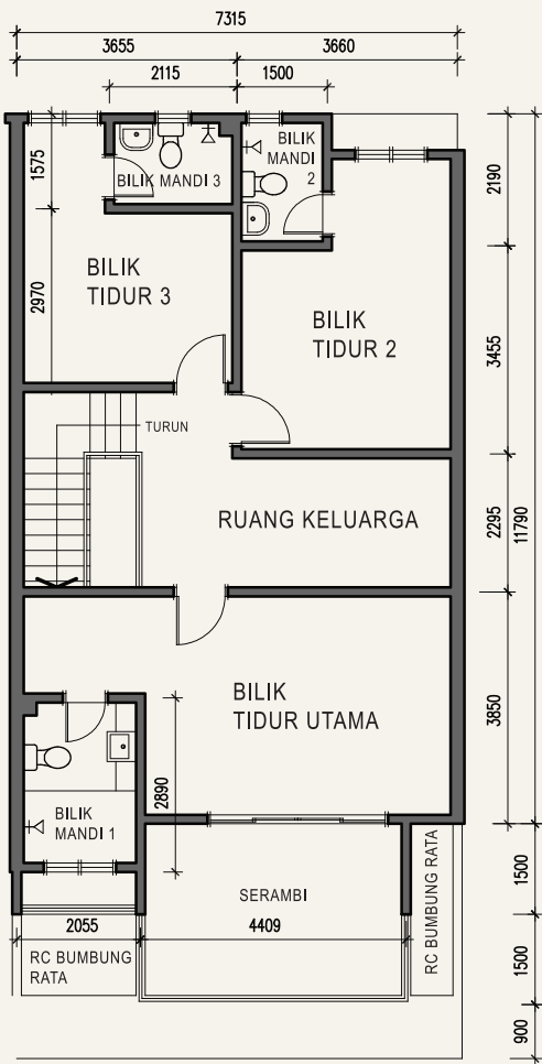
PELAN TINGKAT SATU
