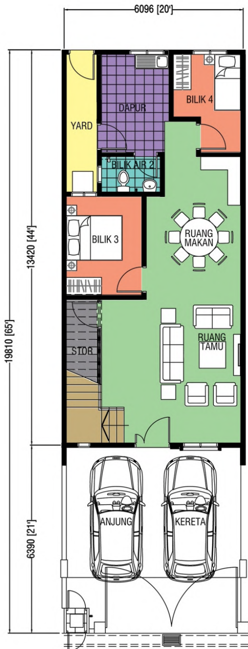
RUMAH TERES 1 ½ TINGKAT (20' X 65') PELAN TINGKAT BAWAH (Lot Tengah)
