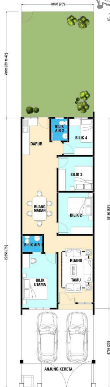
PELAN LANTAI (Lot Tengah) RUMAH TERES SETINGKAT JENIS B (20' x 75')
