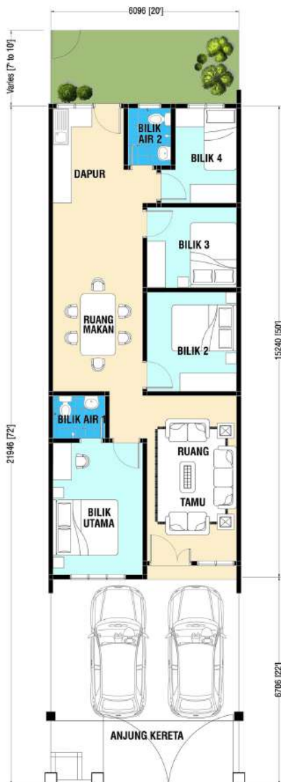
PELAN LANTAI (Lot Tengah) RUMAH TERES SETINGKAT JENIS A (20' x 72')
