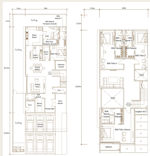
Rumah Berkembar Dua Tingkat Jenis A1
