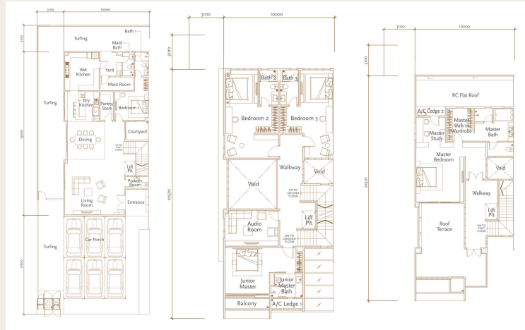
Rumah Berkembar Tiga Tingkat Jenis A
