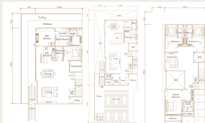
Rumah Berkembar Tiga Tingkat Beserta Aras Bawah Jenis A2
