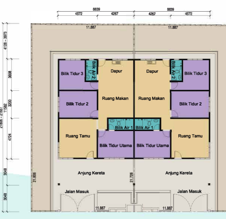
Pelan Tingkat Bawah (Rumah Berkembar 1 Tingkat)
