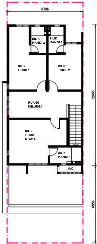
PELAN LANTAI TINGKAT SATU
