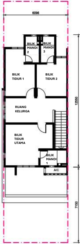
PELAN LANTAI TINGKAT SATU
