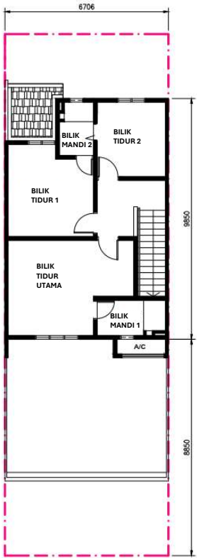
PELAN LANTAI TINGKAT SATU
