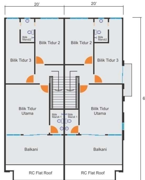
Pelan Lantai Tingkat Atas
