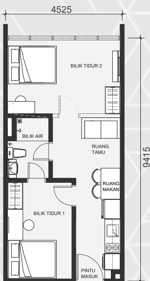
JENIS A 459 Kaki Persegi 2 Bilik Tidur 1 Bilik Air
