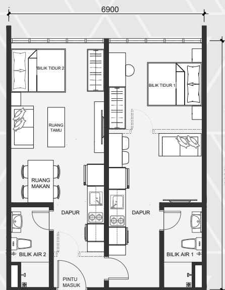
JENIS B 654 Kaki Persegi 2 Bilik Tidur 2 Bilik Air
