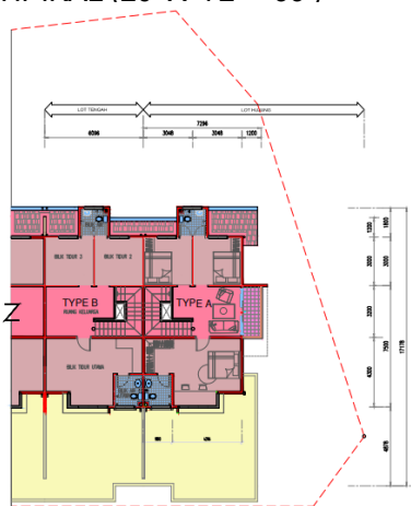
PELAN LANTAI TINGKAT 1 TIPIKAL (20' X 72' – 99')
