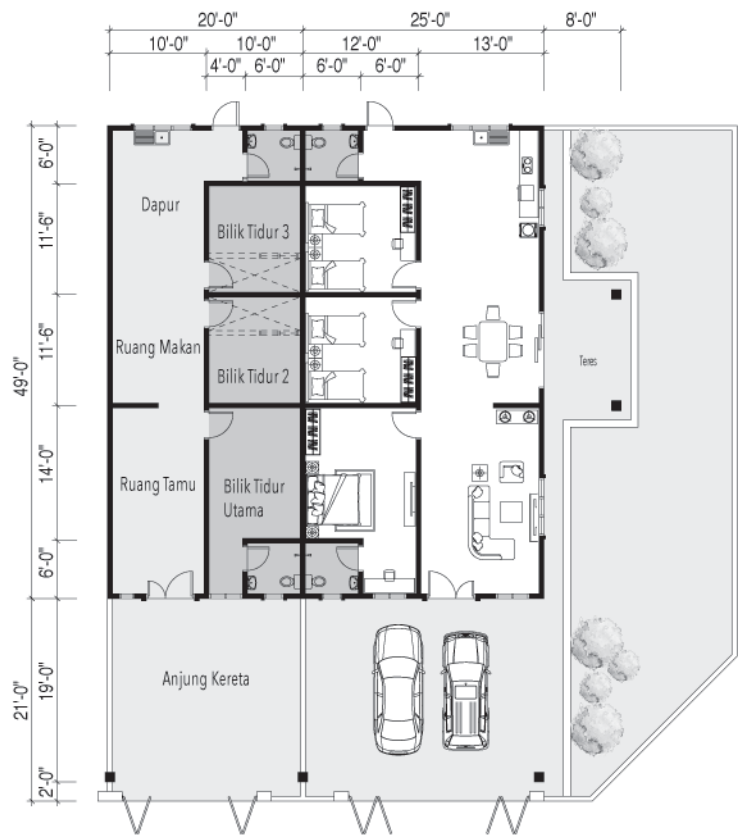
25'x70' (Jenis A)
