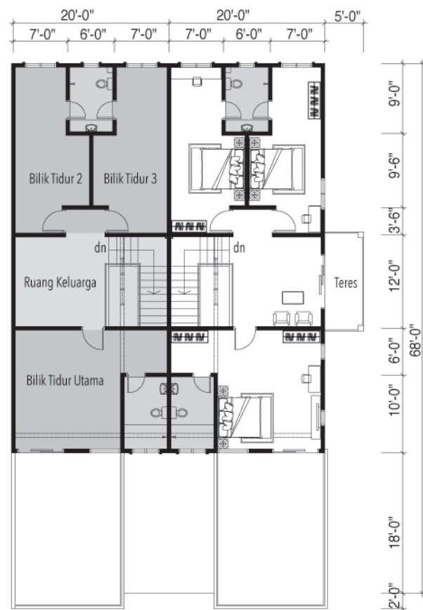
PELAN TINGKAT ATAS
