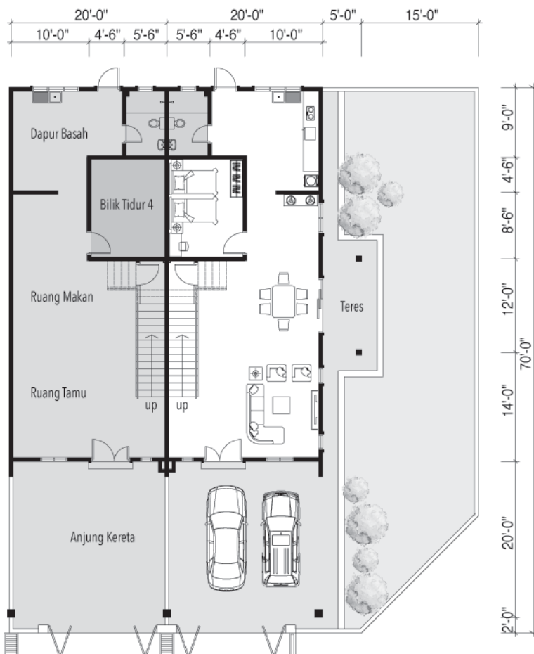
PELAN TINGKAT BAWAH
