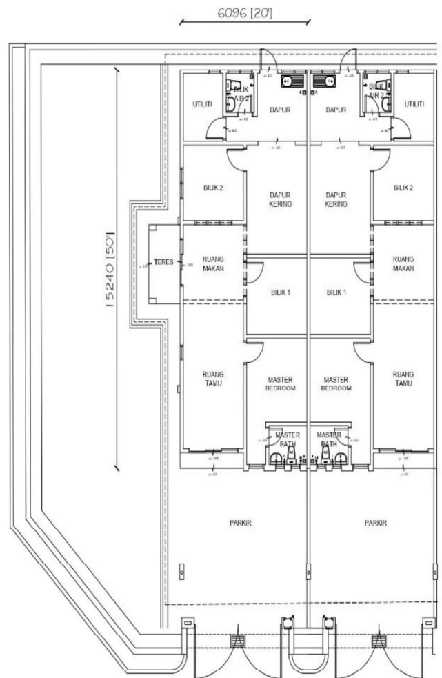
Pelan Lantai
