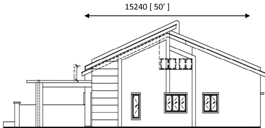
Pandangan Belakang
