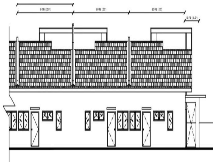
Pandangan Belakang
