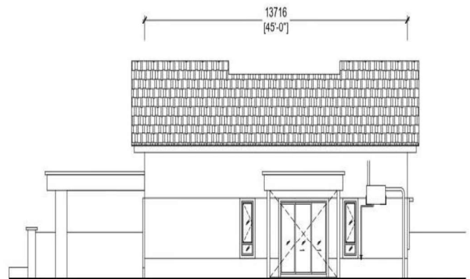
Pandangan Sisi Kiri
