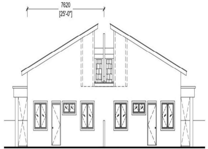
Pandangan Belakang
