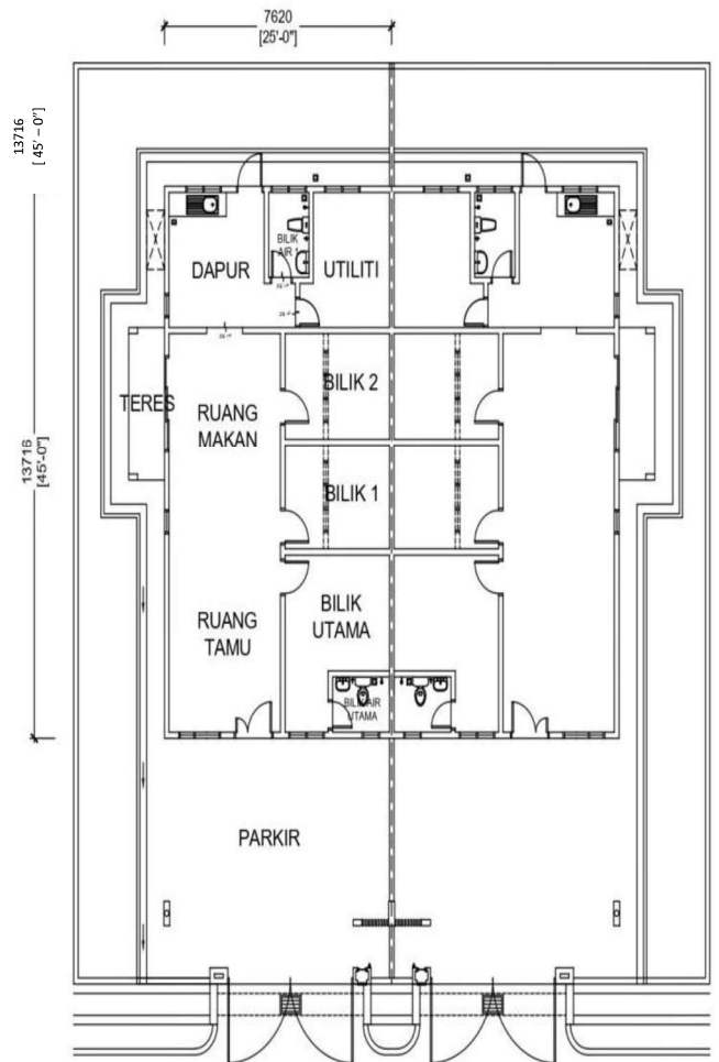
Pelan Lantai
