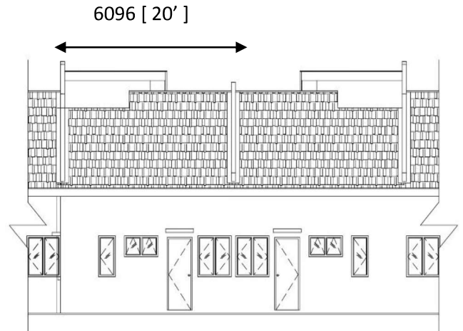
Pandangan Belakang
