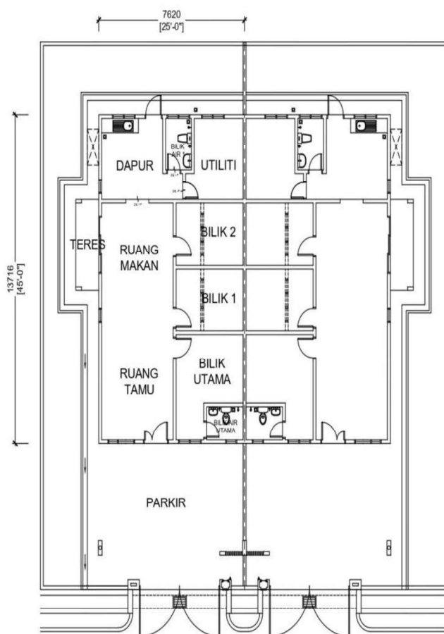
Pelan Lantai
