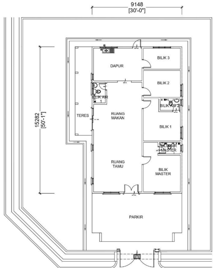
Pelan Lantai
