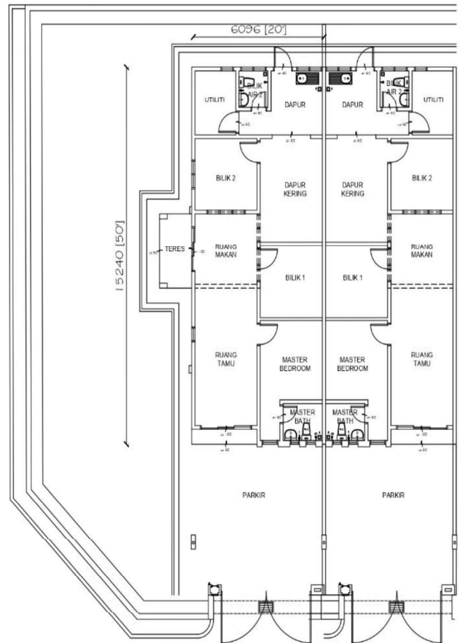
Pelan Lantai
