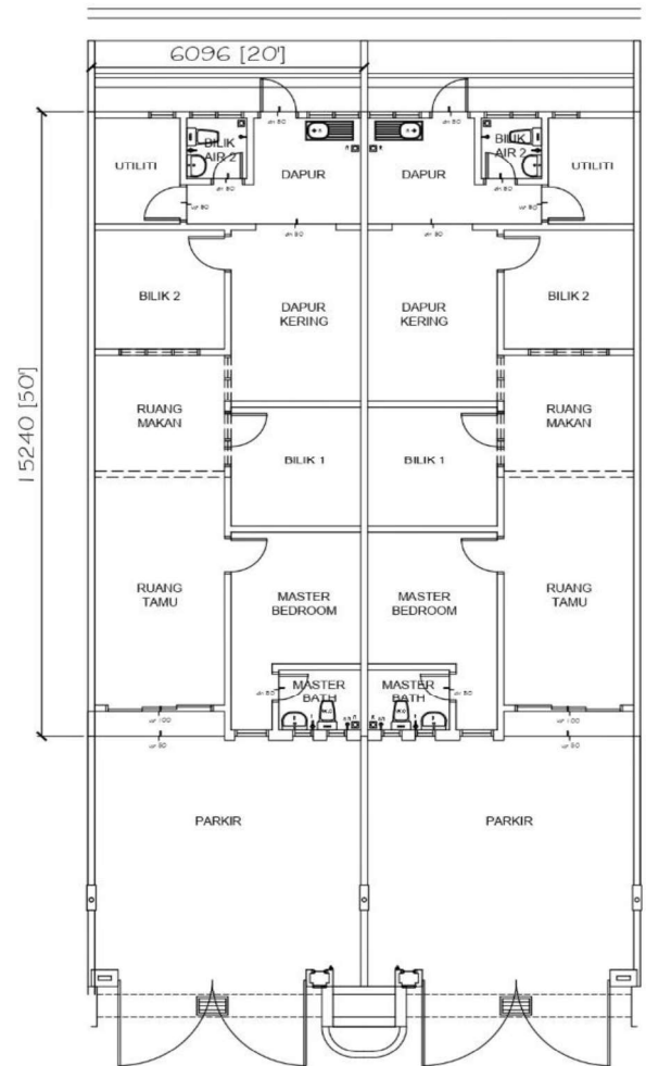
Pelan Lantai
