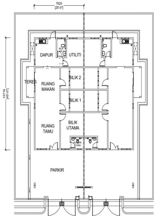
Pelan Lantai
