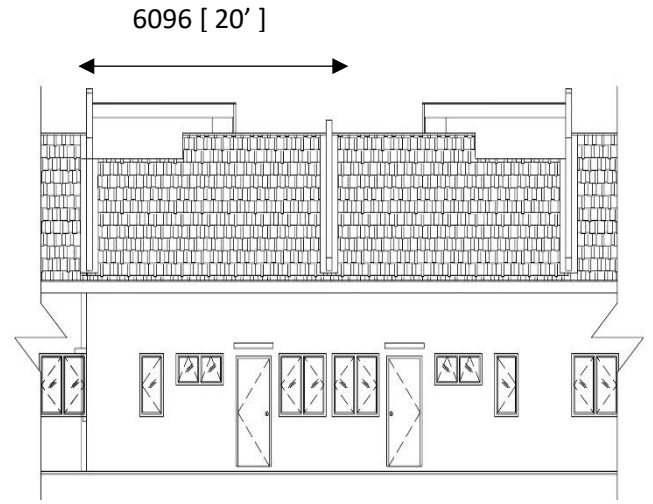
Pandangan Belakang
