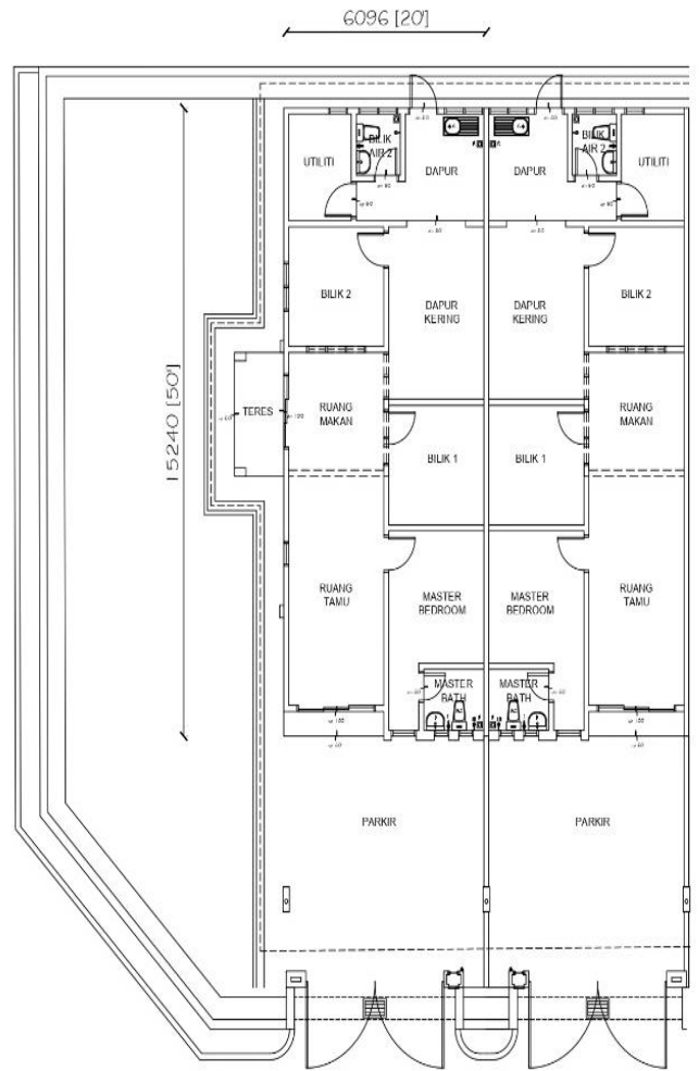
Pelan Lantai
