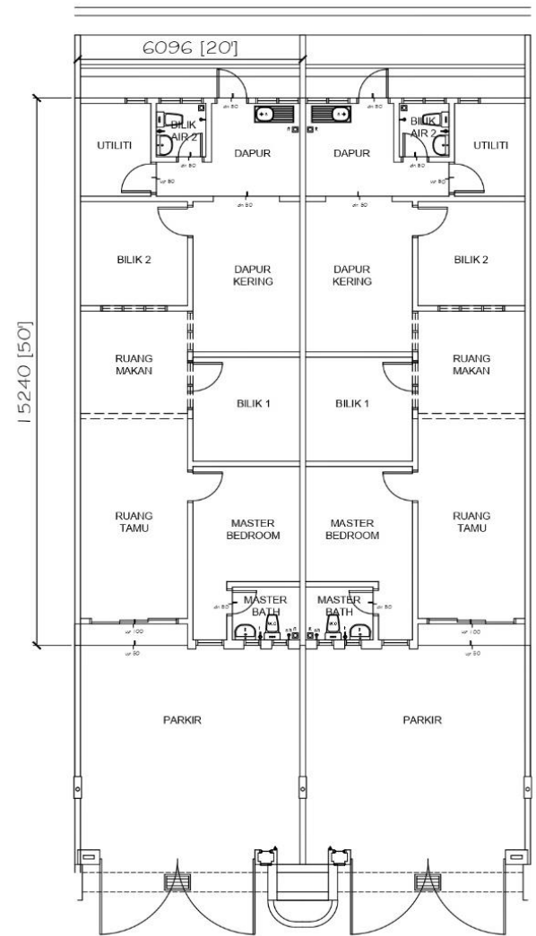
Pelan Lantai
