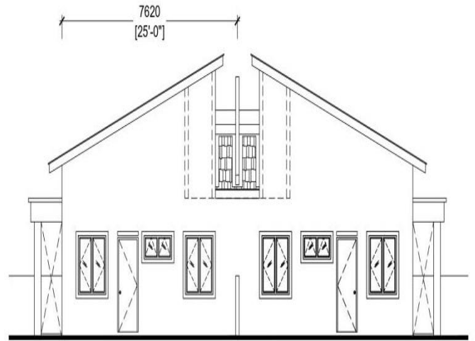
Pandangan Belakang
