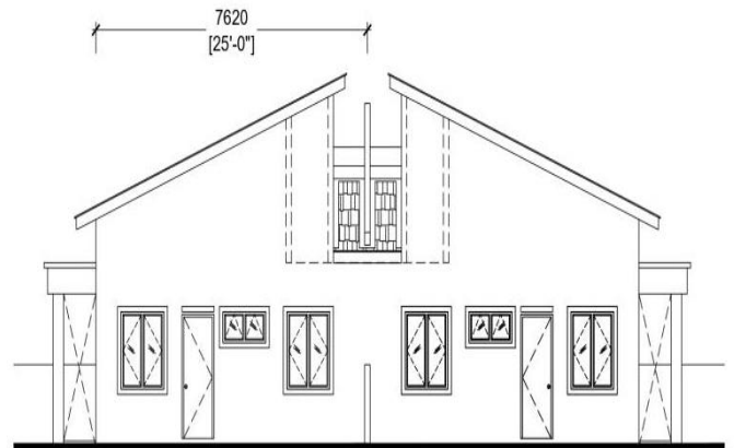
Pandangan Belakang
