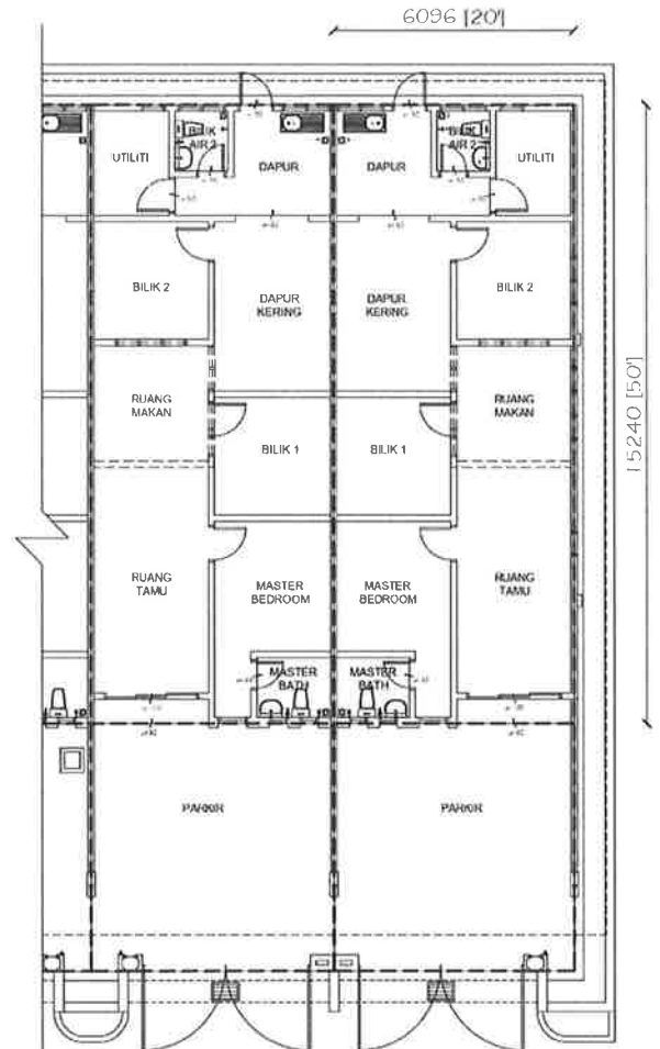
Pelan Lantai
