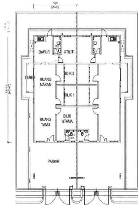
Pelan Lantai
