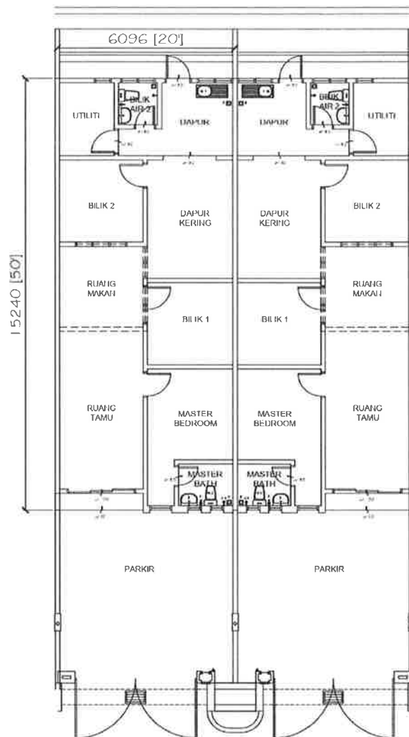
Pelan Lantai
