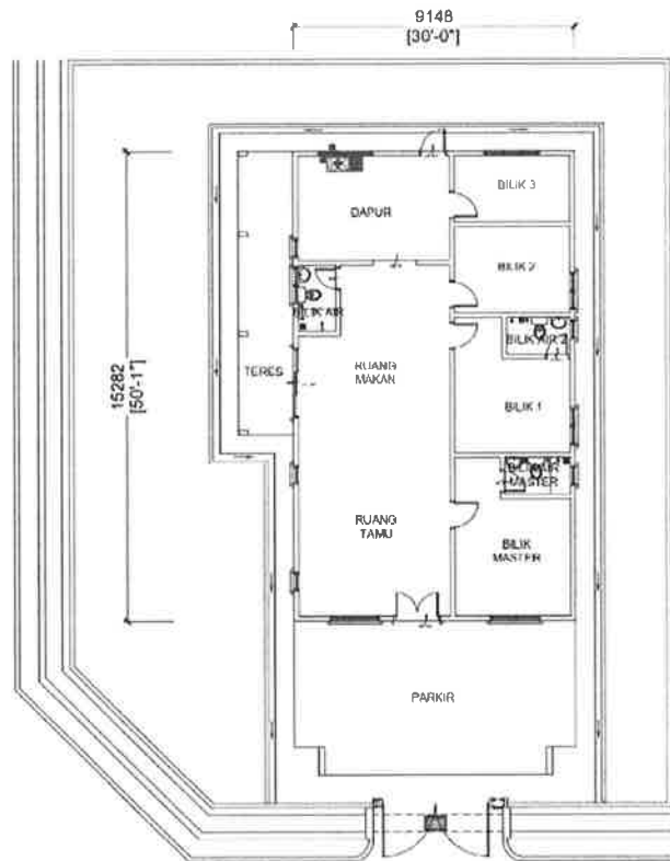
Pelan Lantai
