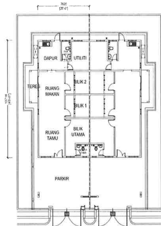
Pelan Lantai
