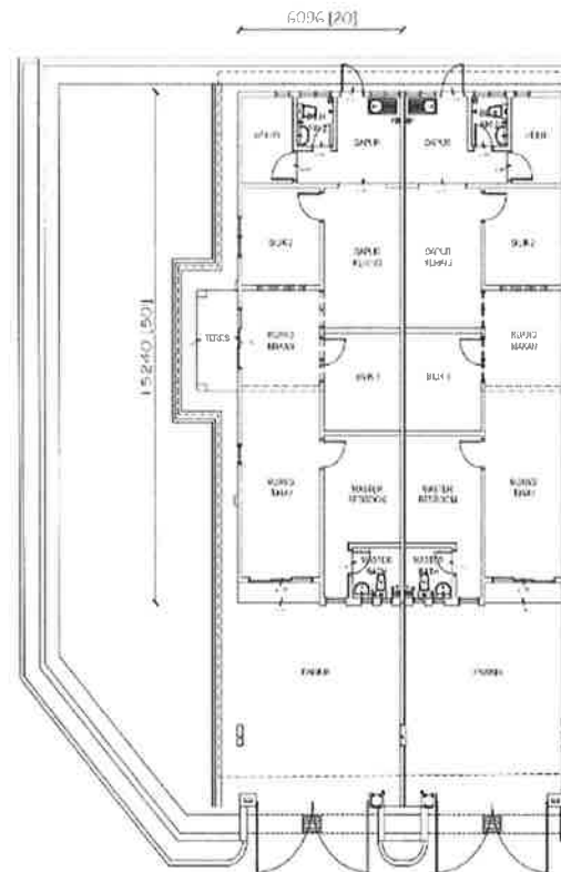
Pelan Lantai
