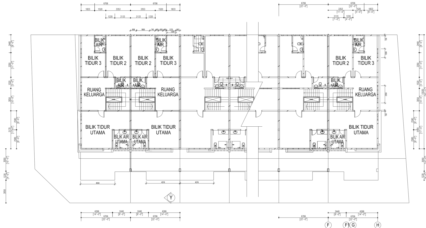
PELAN LANTAI - TINGKAT SATU
