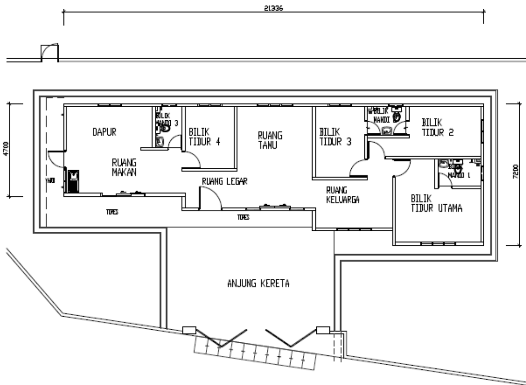
PELAN LANTAI TINGKAT BAWAH
