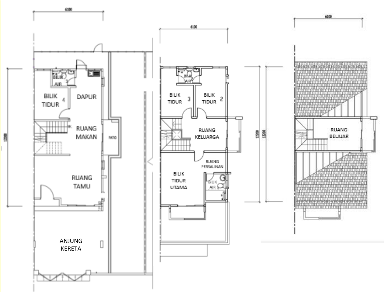
PELAN LANTAI TINGKAT BAWAH PELAN LANTAI TINGKAT SATU PELAN LANTAI TINGKAT DUA
