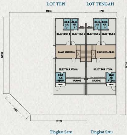
Jenis C 22' x 70' Keluasan Binaan: 2,203 kps. 4 Bilik Tidur 4 Bilik Air
