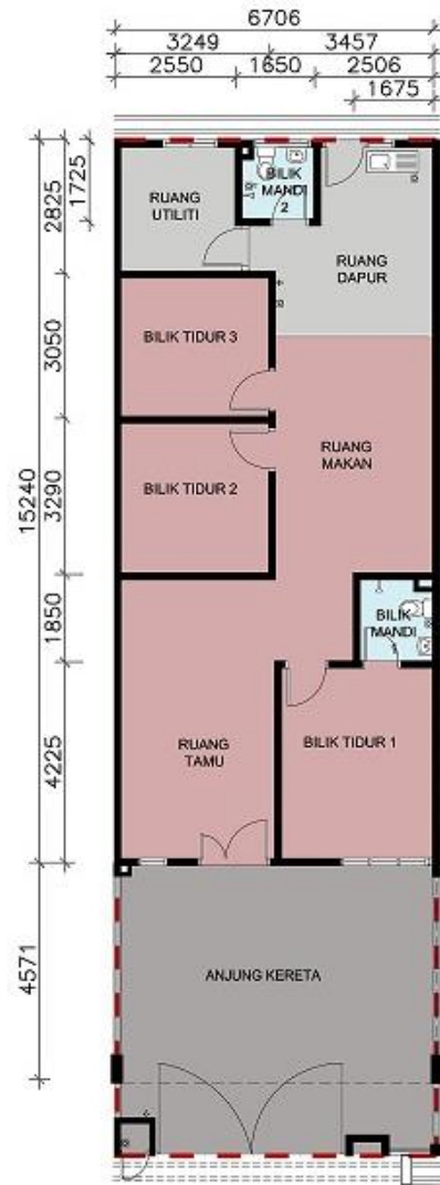
Rumah Teres 1 Tingkat 22' x 70' & 22' x 66'
