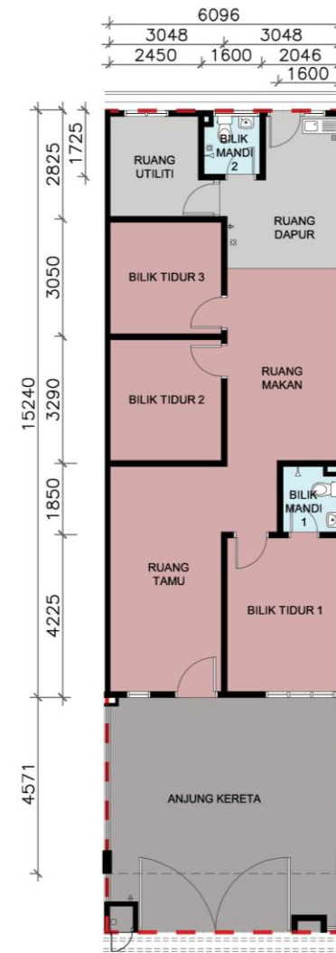
Rumah Teres Mampu Milik 1 Tingkat 20' x 70'
