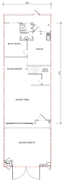
PELAN TINGKAT BAWAH
