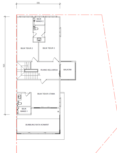
PELAN TINGKAT ATAS
