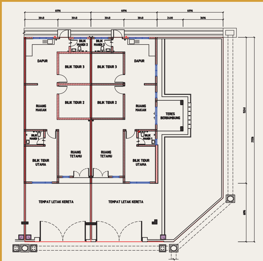
Pelan Tingkat Aras Tanah
