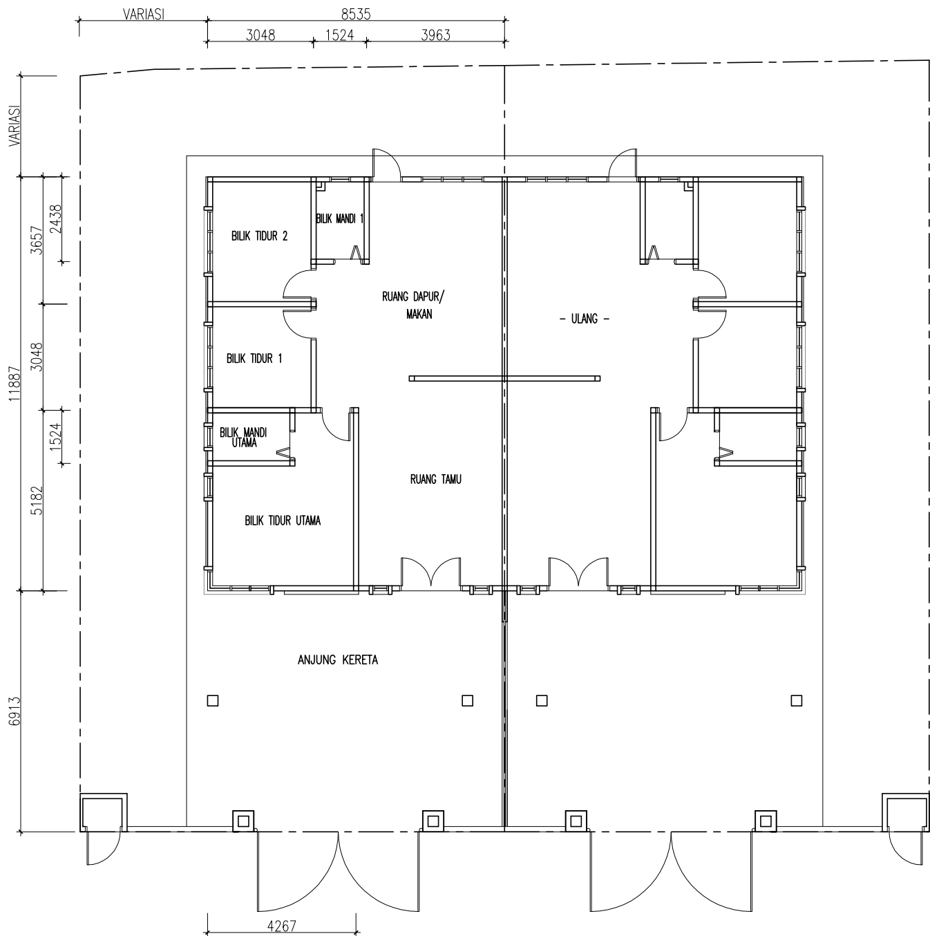
PELAN LANTAI ARAS BAWAH
