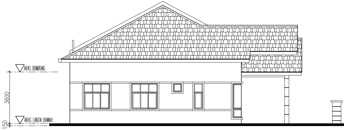
PANDANGAN SISI
