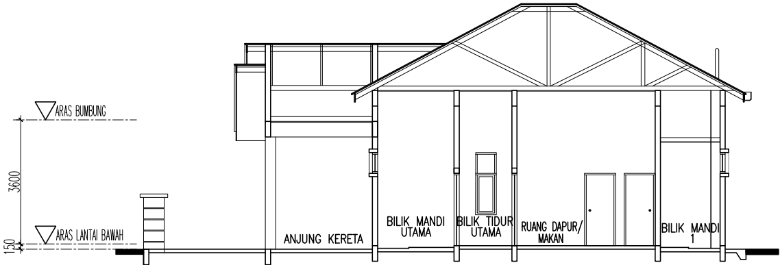
KERATAN
