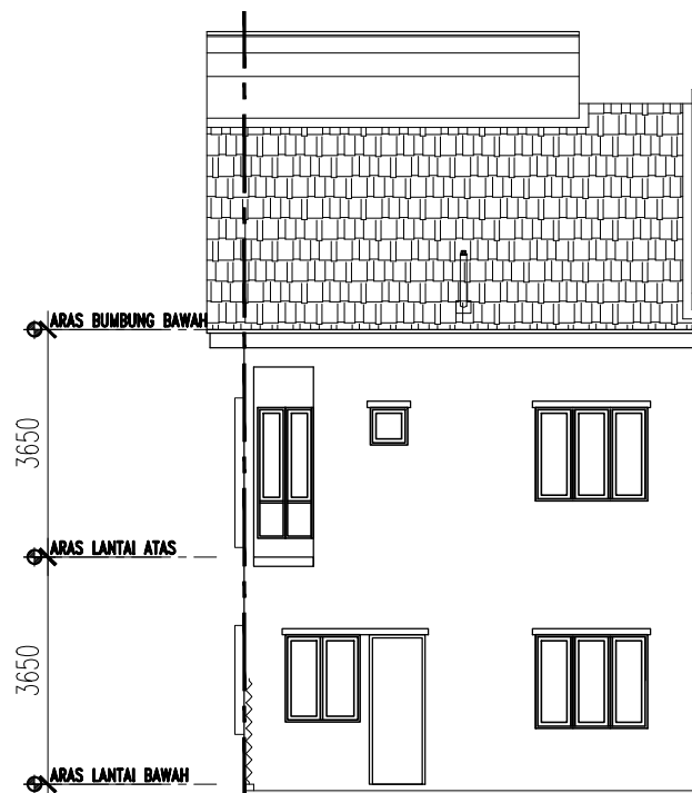
PANDANGAN BELAKANG
