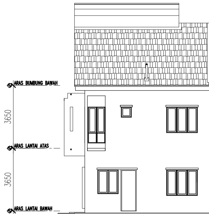
PANDANGAN BELAKANG
