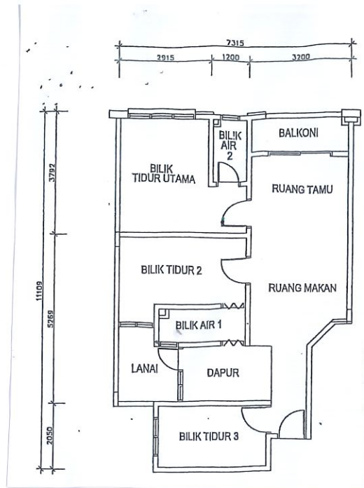
TYPE H1 : 70.88 meter persegi
