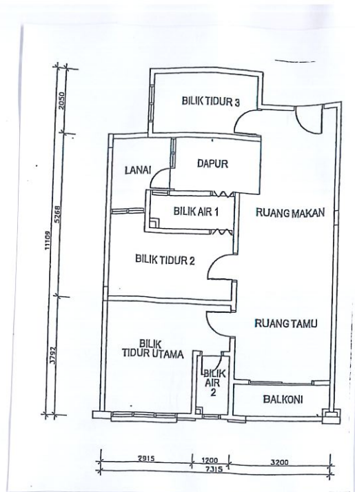
TYPE H3 : 75.06 meter persegi
