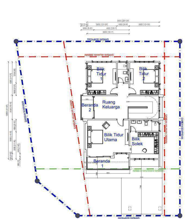
Pelan Lantai Tingkat 1
