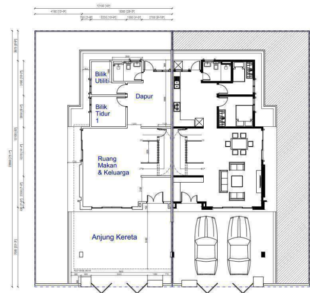
Pelan Lantai Tingkat 1 Rumah Berkembar 2 Tingkat
