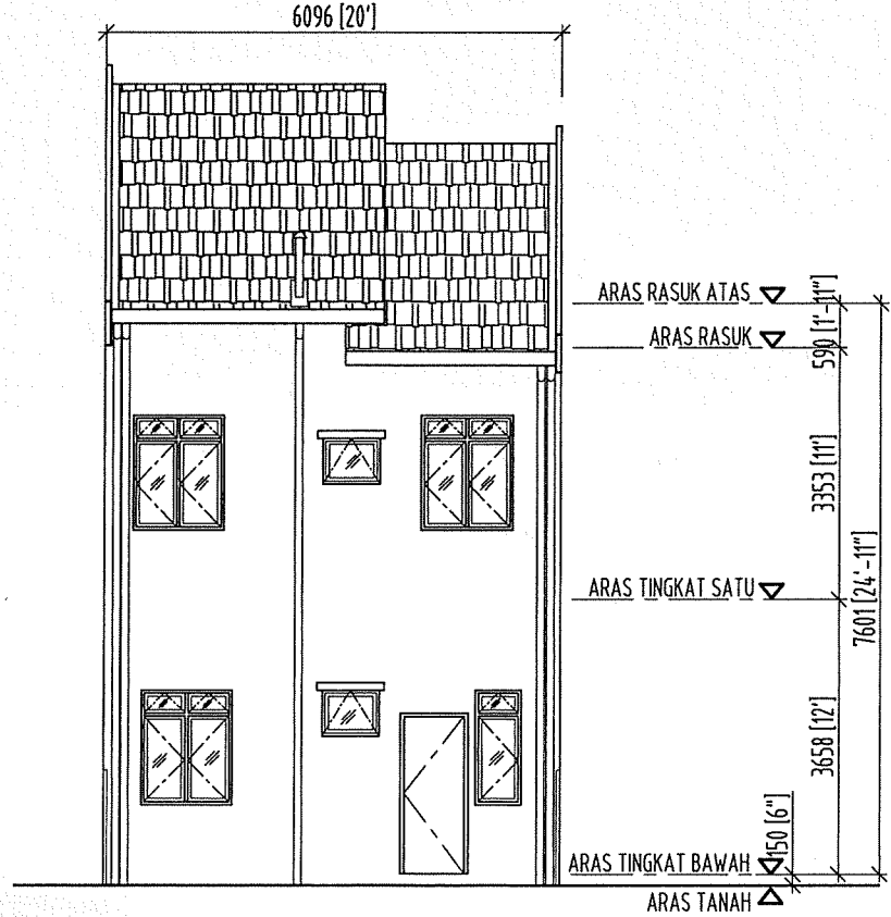
PANDANGAN BELAKANG
