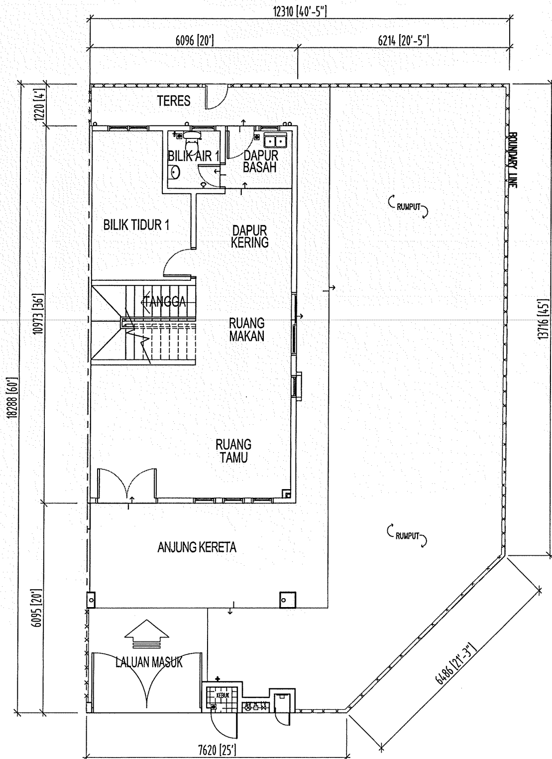
PELAN LANTAI TINGKAT BAWAH
