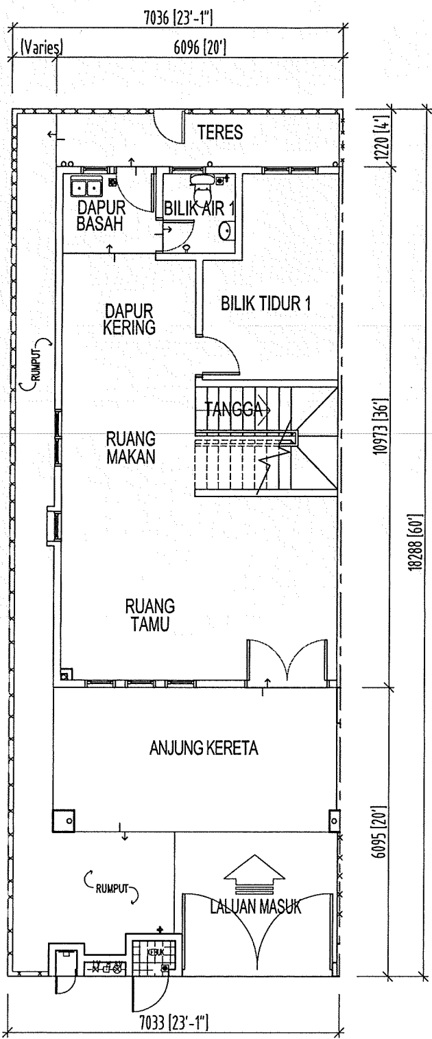
PELAN LANTAI TINGKAT BAWAH
