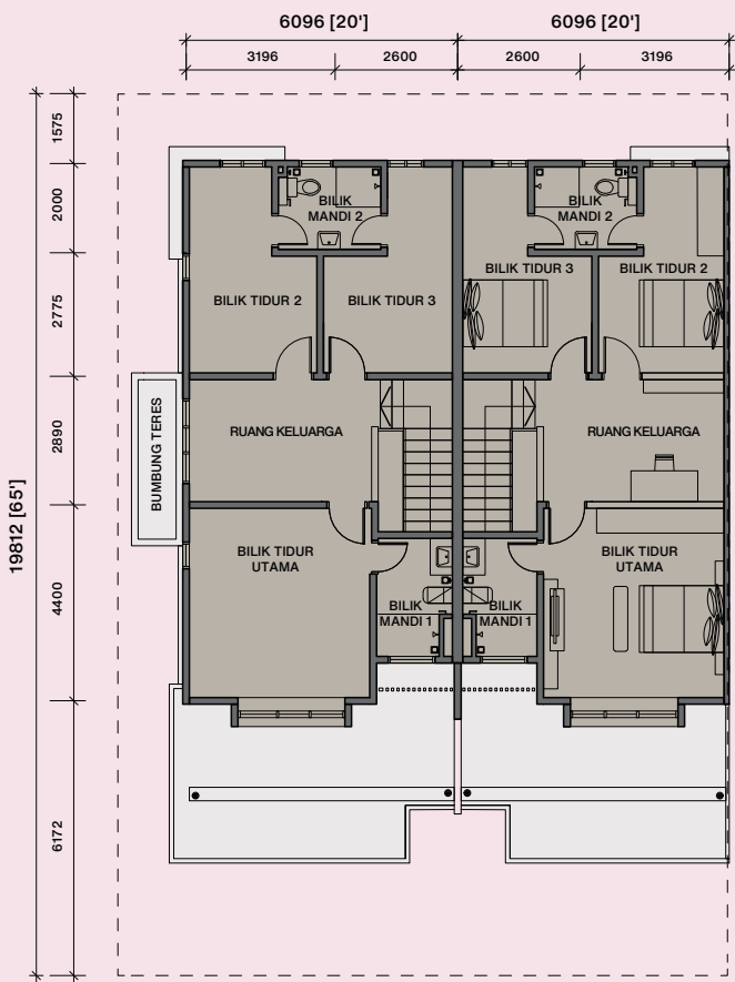
Tingkat Atas
