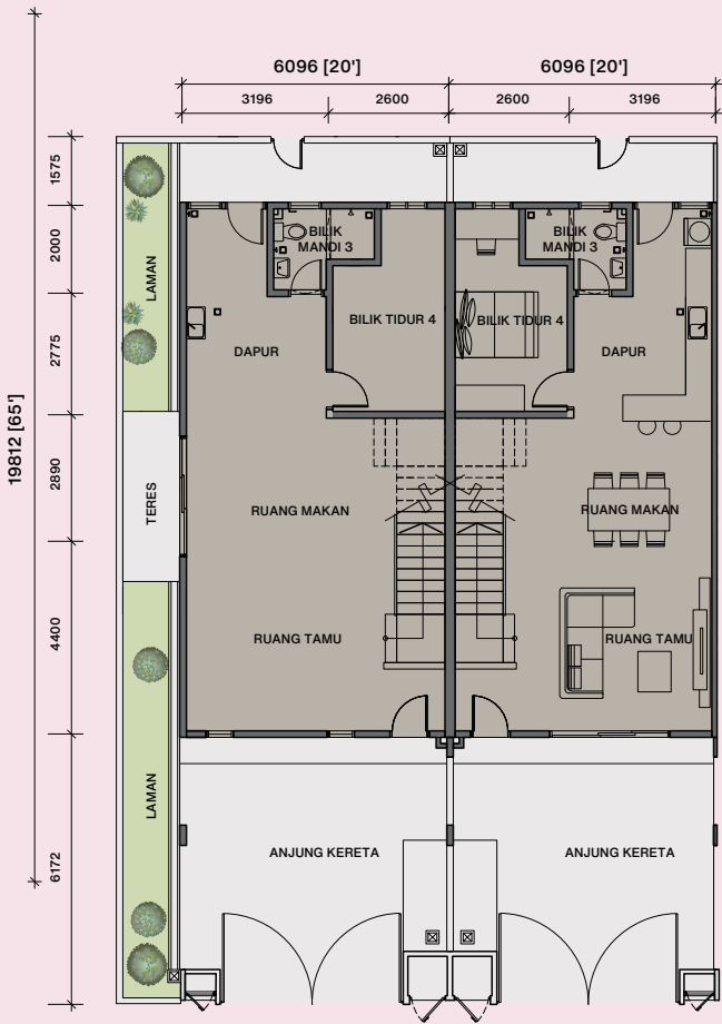
Tingkat Bawah
