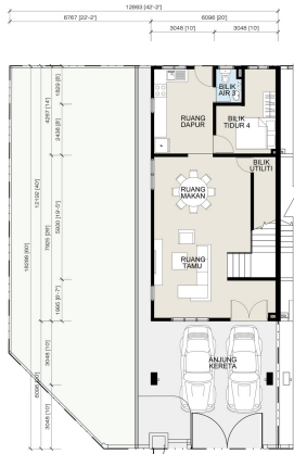
PELAN TINGKAT BAWAH Unit Sudut
