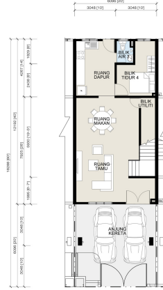
PELAN TINGKAT BAWAH Unit Tengah
