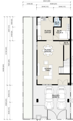
PELAN TINGKAT BAWAH Unit Hujung
