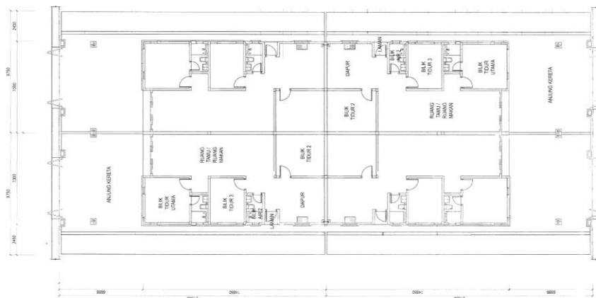
Pelan Lantai Rumah Kluster 1 Tingkat (Jenis B)
