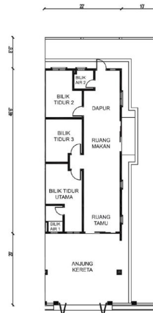
Pelan Lantai
