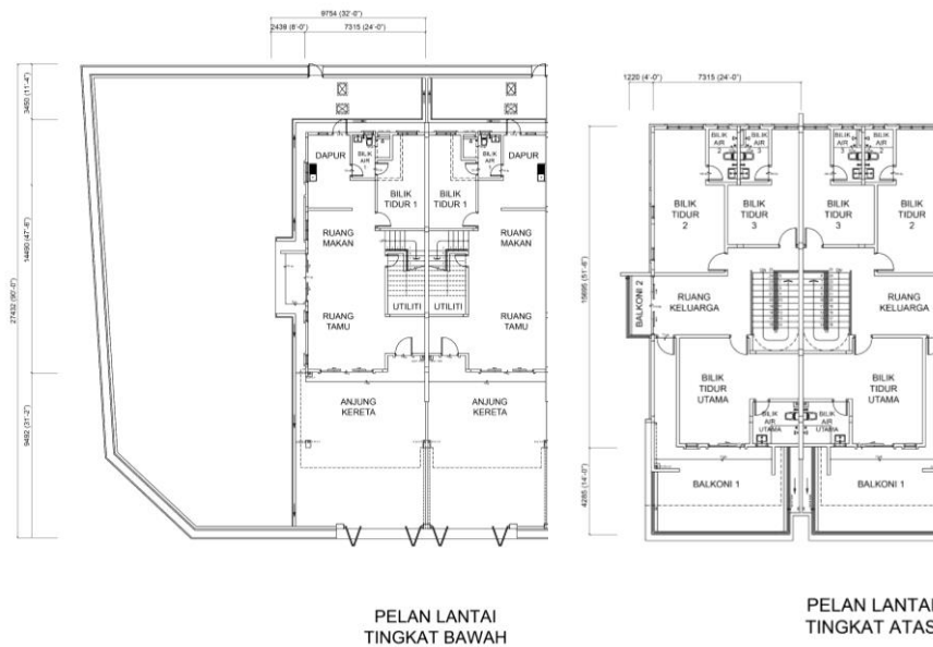
Pelan Lantai
