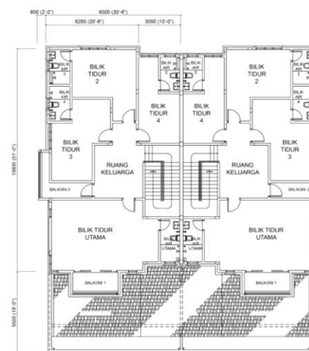
PELAN LANTAI TINGKAT ATAS
