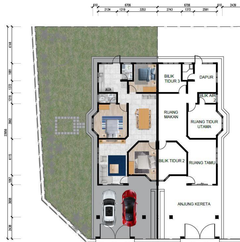
PELAN LANTAI TYPE A
