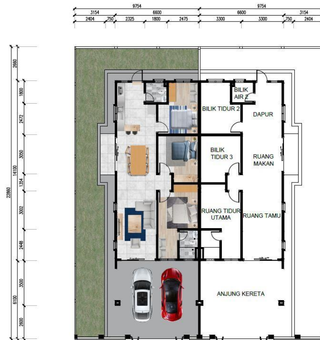
PELAN LANTAI TYPE B
