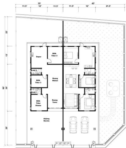
Pelan Lantai
