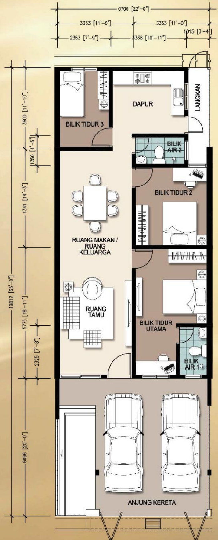
PELAN LANTAI
