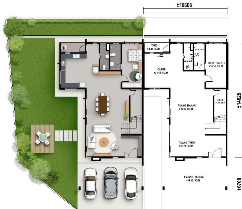
PELAN LANTAI TINGKAT BAWAH RUMAH TERES 2-TINGKAT
