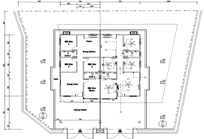
PELAN LANTAI
