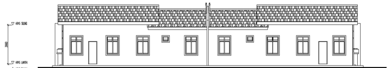
PANDANGAN BELAKANG
