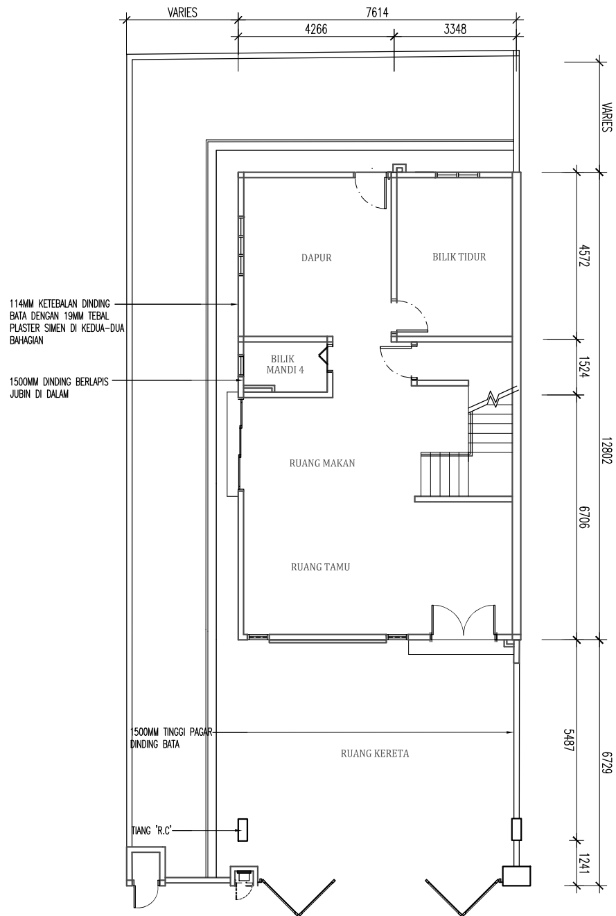
PELAN LANTAI TINGKAT BAWAH
