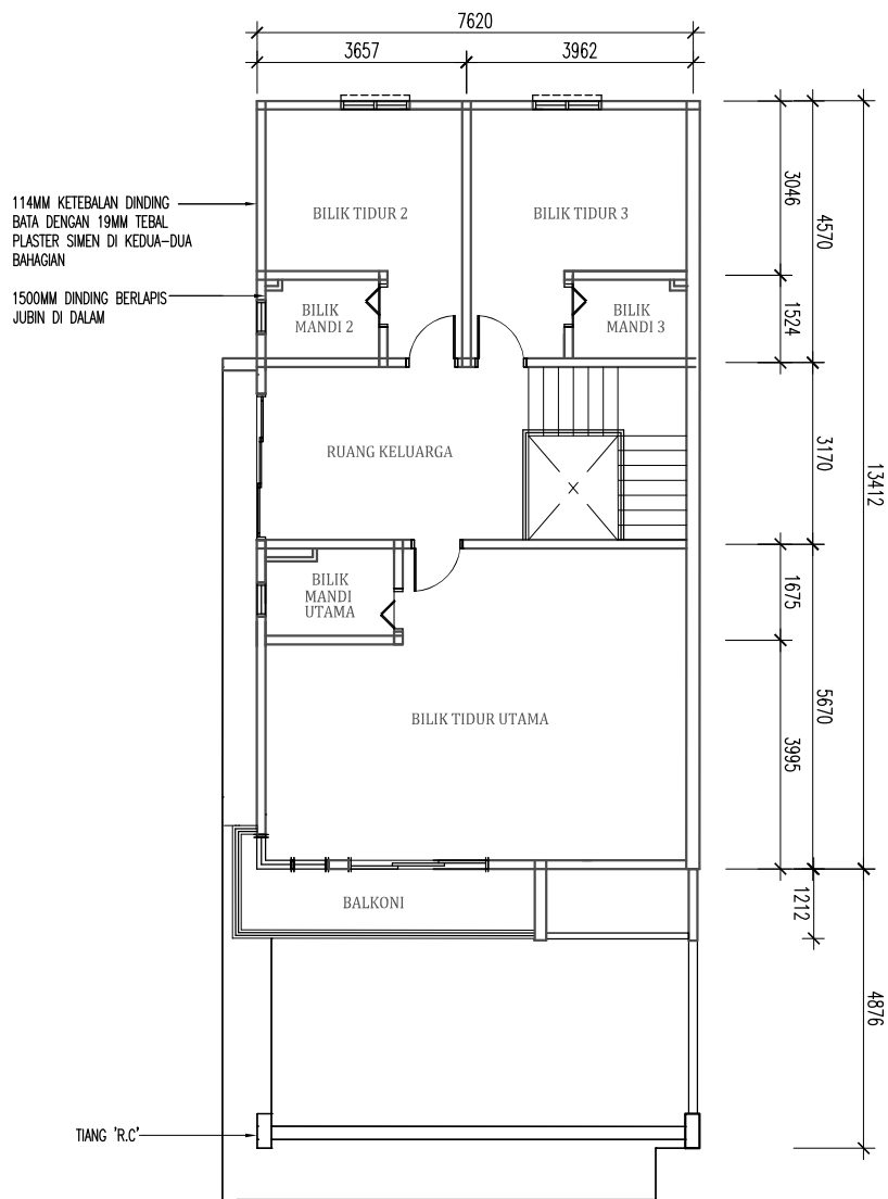
PELAN LANTAI TINGKAT KEDUA
