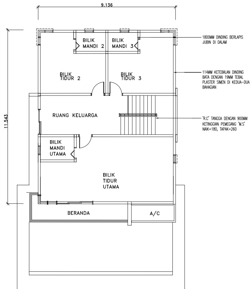
PELAN ARAS SATU
