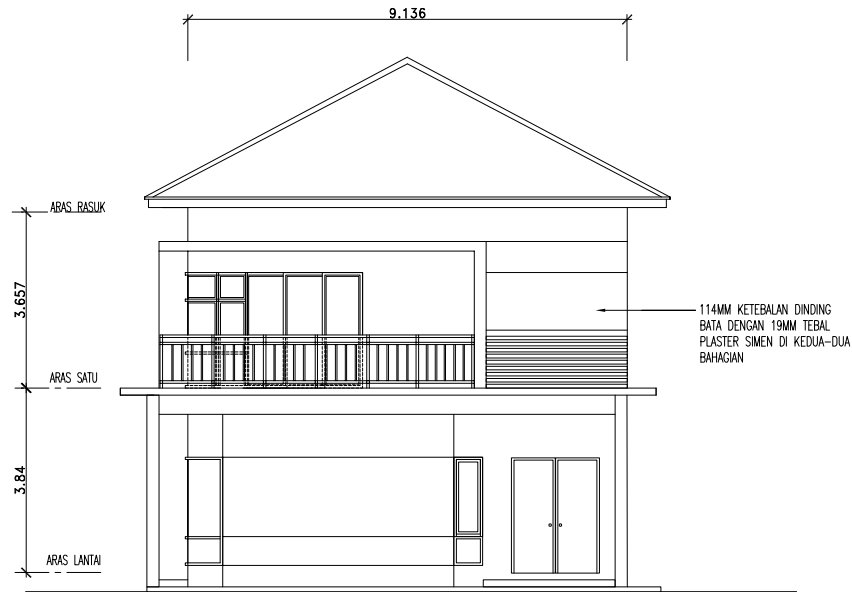
PANDANGAN DEPAN
