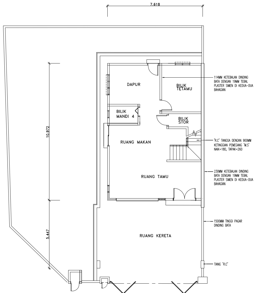
PELAN LANTAI
