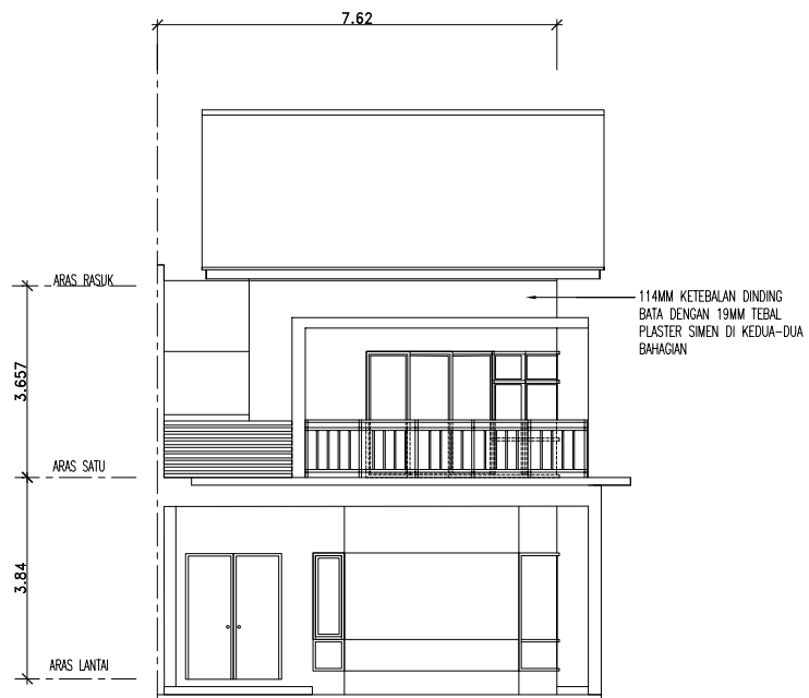
PANDANGAN DEPAN
