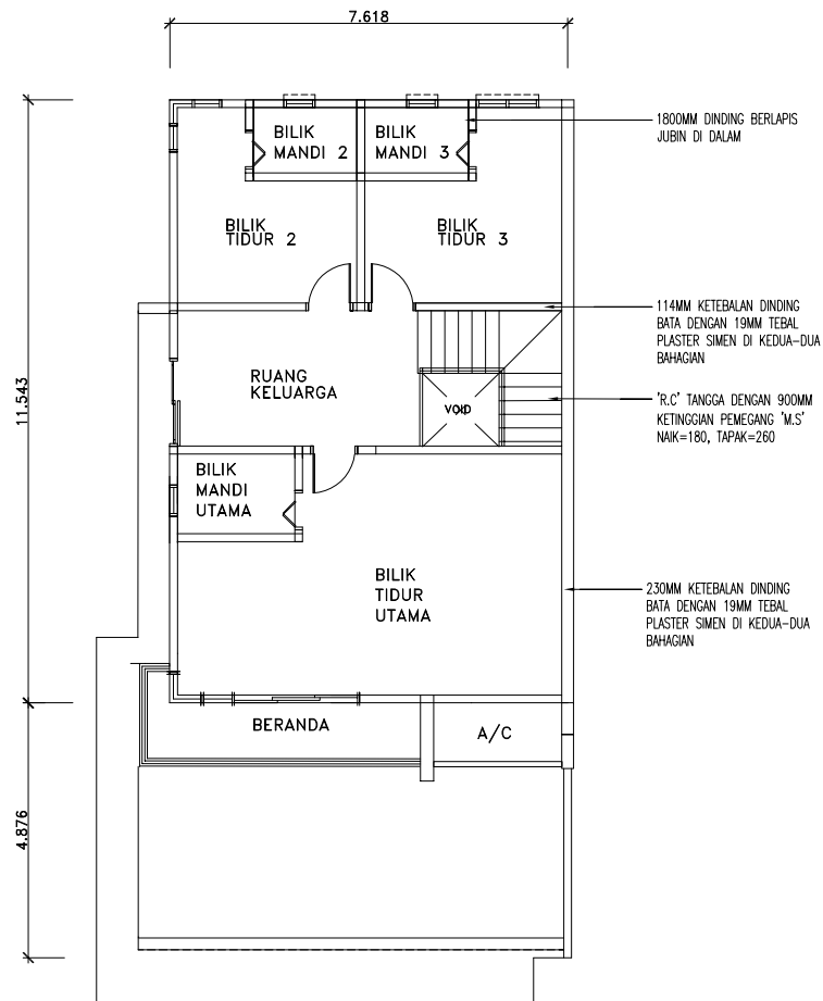
PELAN ARAS SATU
