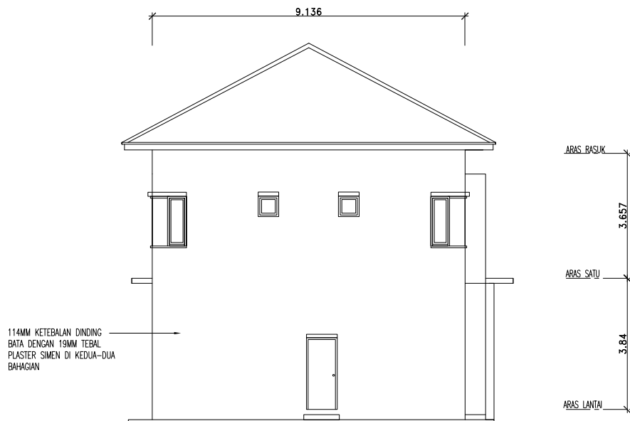
PANDANGAN BELAKANG
