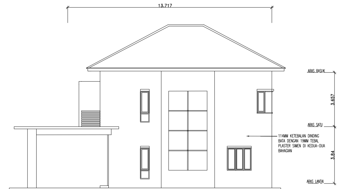
PANDANGAN KANAN
