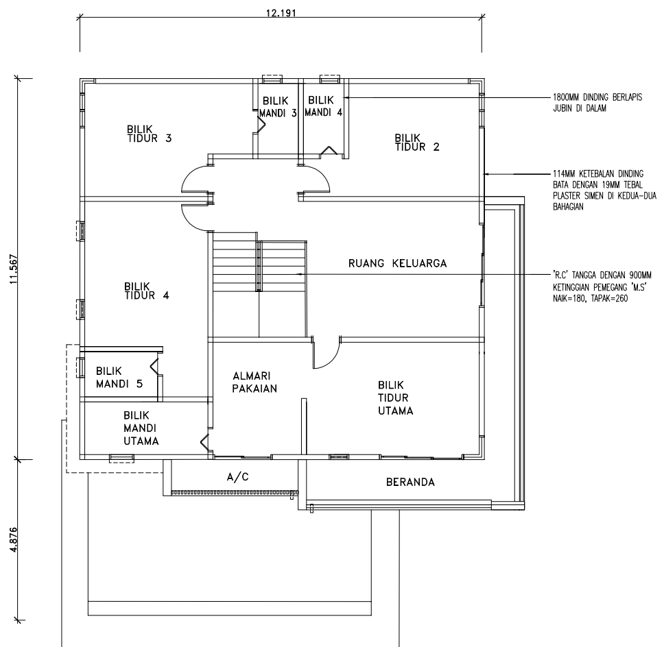
PELAN ARAS SATU
