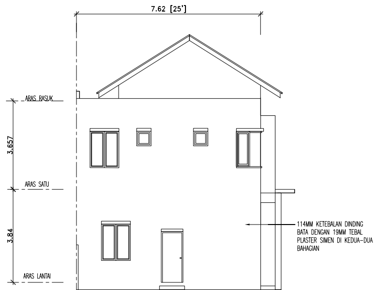
PANDANGAN BELAKANG
