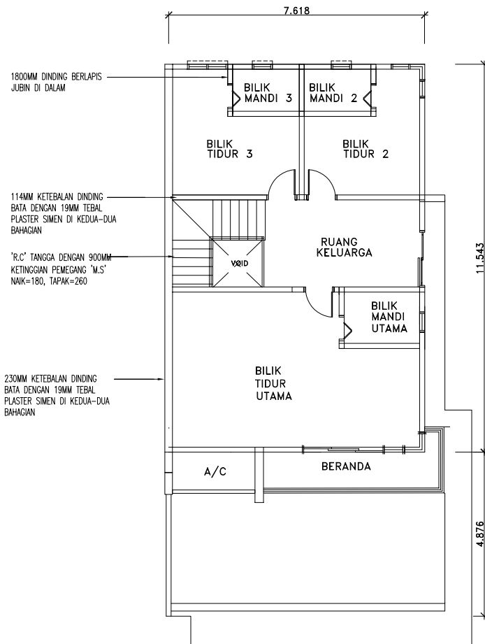
PELAN ARAS SATU
