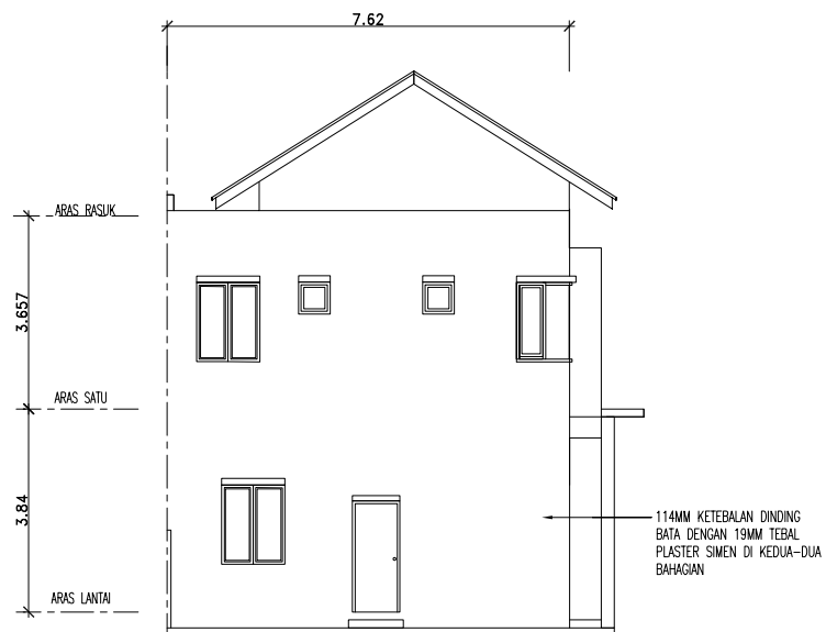
PANDANGAN BELAKANG
