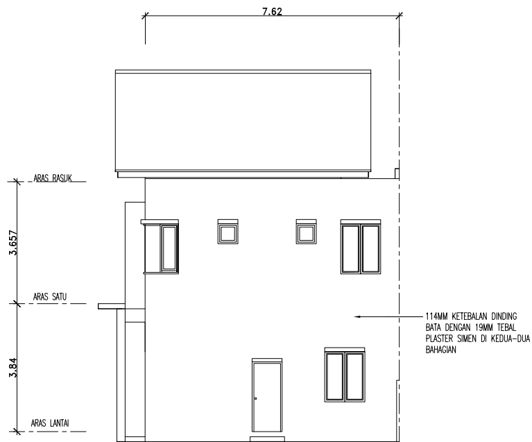
PANDANGAN BELAKANG
