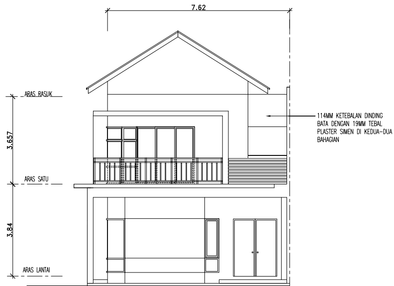
PANDANGAN DEPAN
