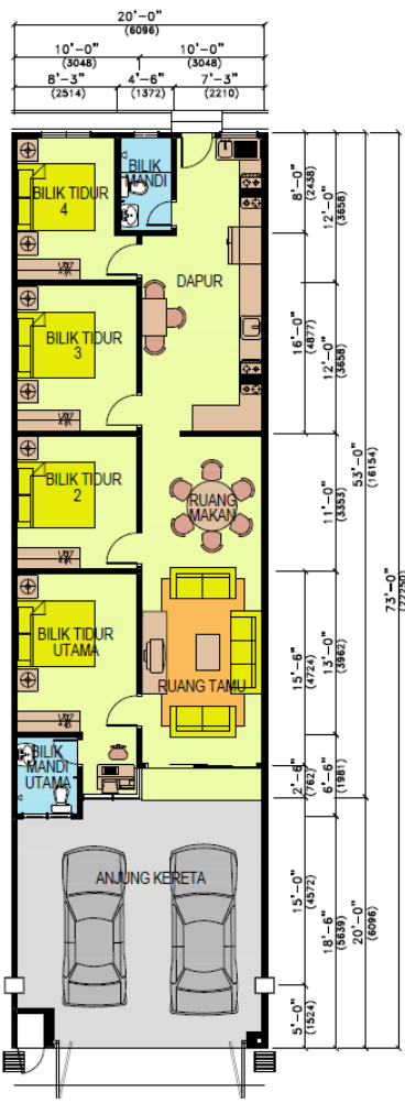
PELAN LANTAI
