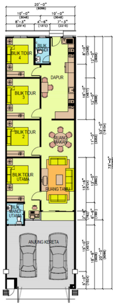
PELAN LANTAI
