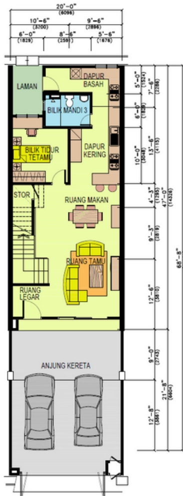
PELAN TINGKAT BAWAH
