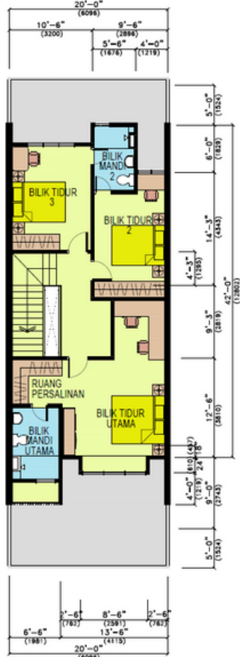
PELAN TINGKAT ATAS
