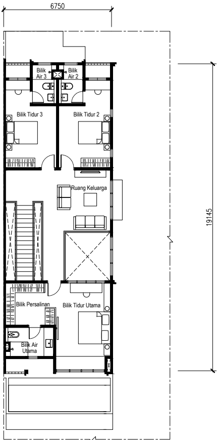
Pelan Lantai Tingkat 1
