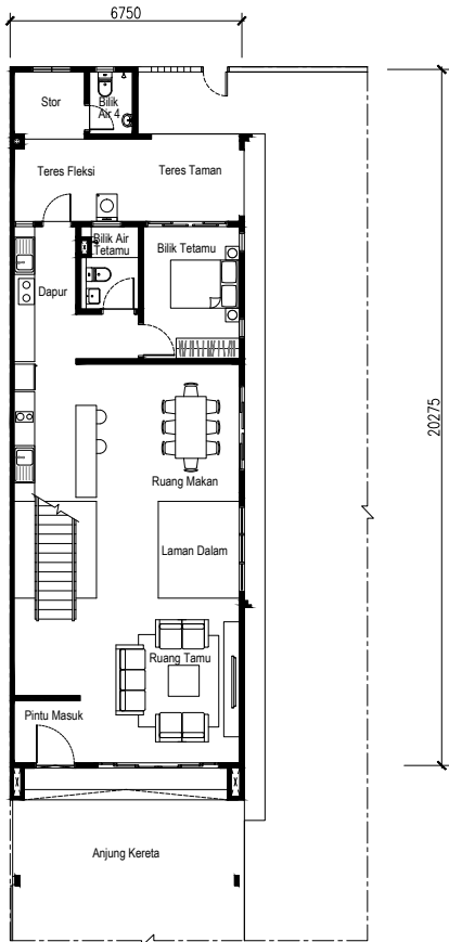
Pelan Lantai Bawah
