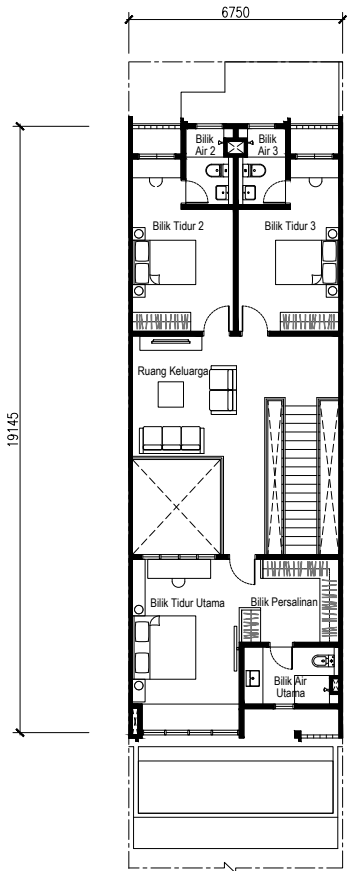
Pelan Lantai Tingkat 1
