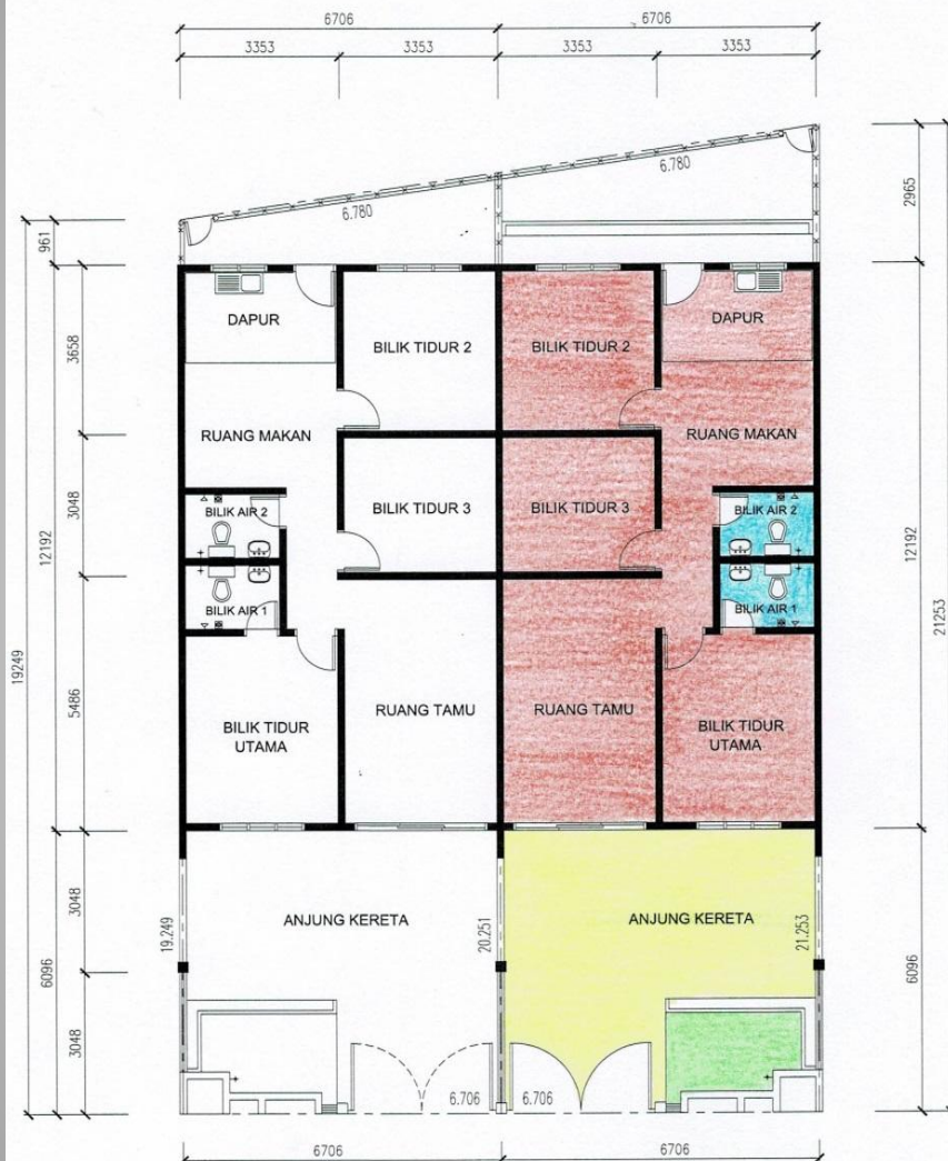
PELAN ARAS TINGKAT BAWAH scale 1: 100
