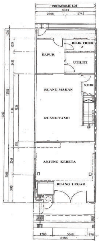
PELAN TINGKAT BAWAH
