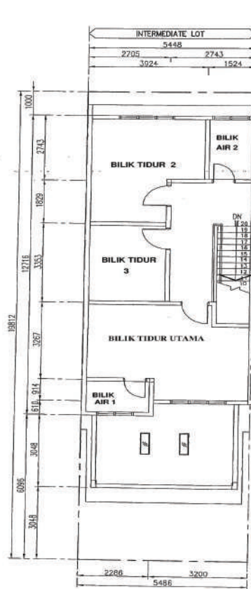
PELAN TINGKAT SATU
