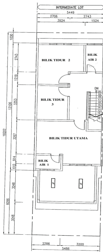
PELAN TINGKAT SATU
