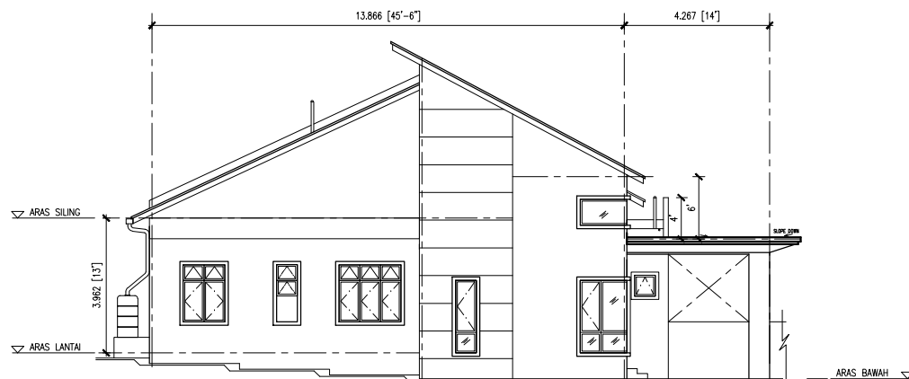
PANDANGAN SISI RUMAH BERBANDUNG SATU TINGKAT
