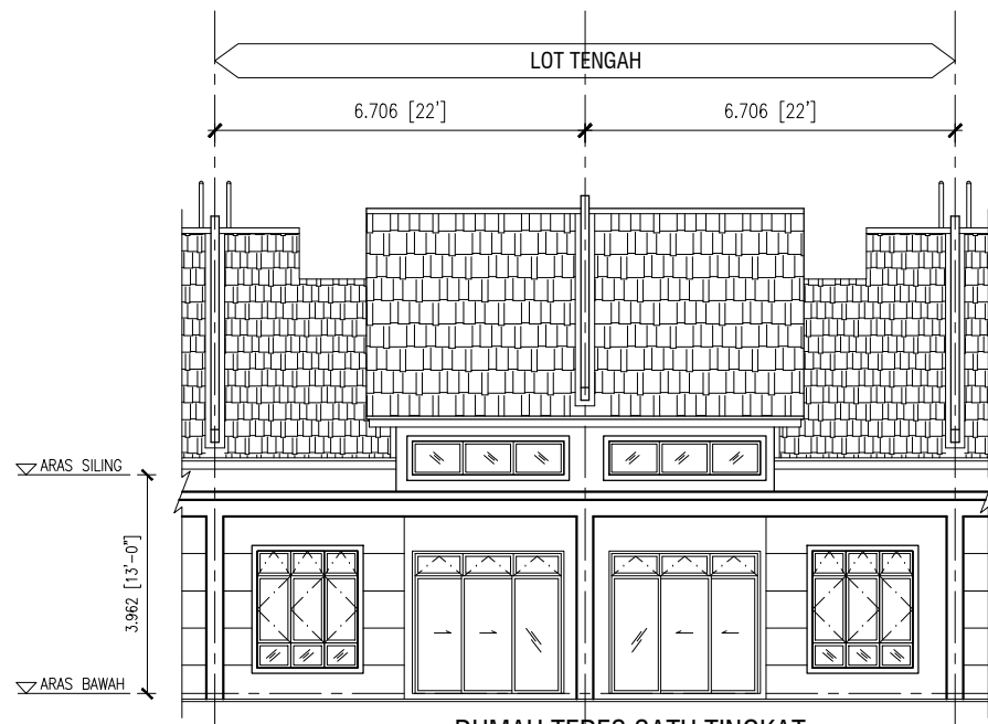
RUMAH TERES SATU TINGKAT PANDANGAN HADAPAN
