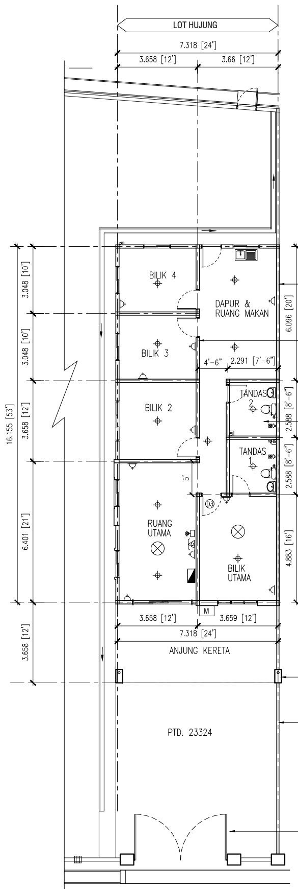
RUMAH TERES SATU TINGKAT PELAN LANTAI KELUASAN LANTAI: 118.23m 2
