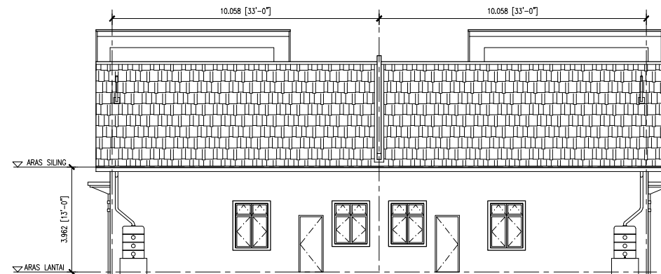
PANDANGAN BELAKANG
