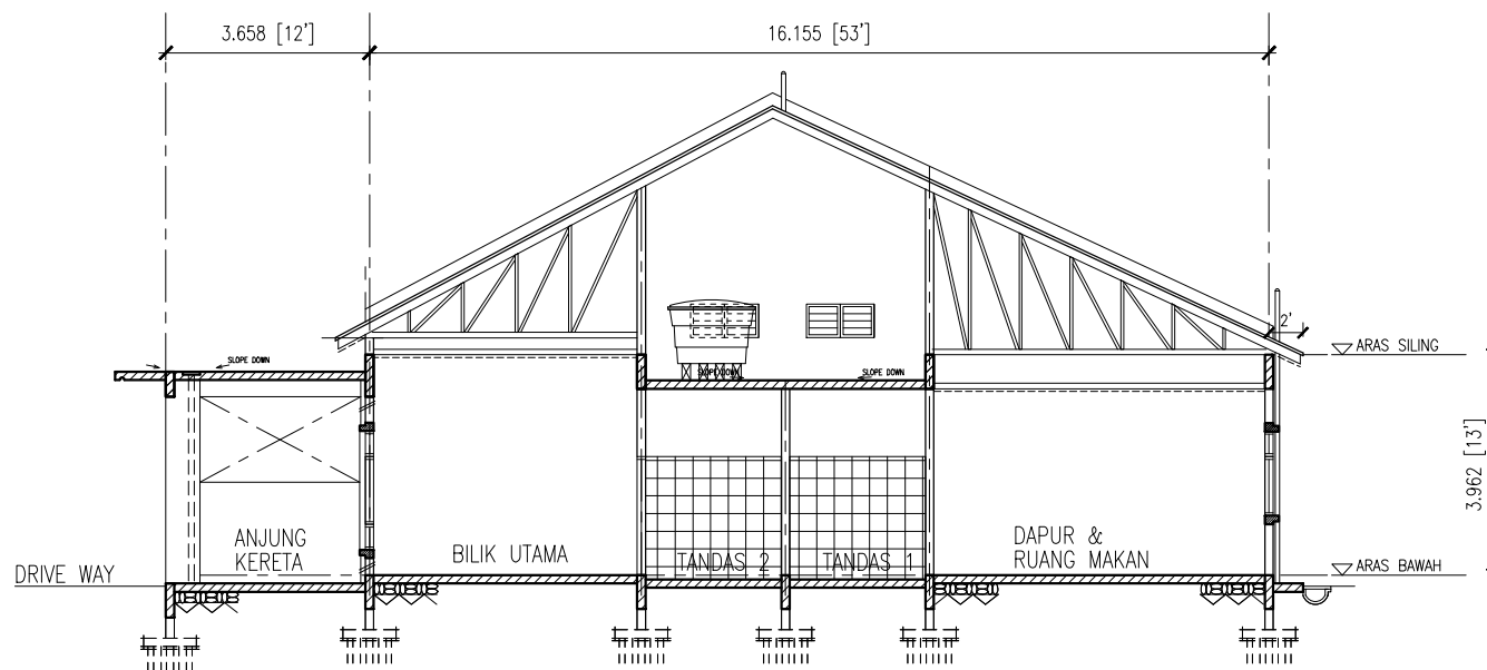
KERATAN R-R
