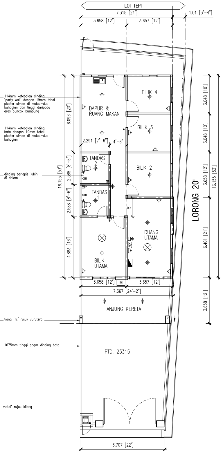
RUMAH TERES SATU TINGKAT PELAN LANTAI KELUASAN LANTAI: 118.17m 2
