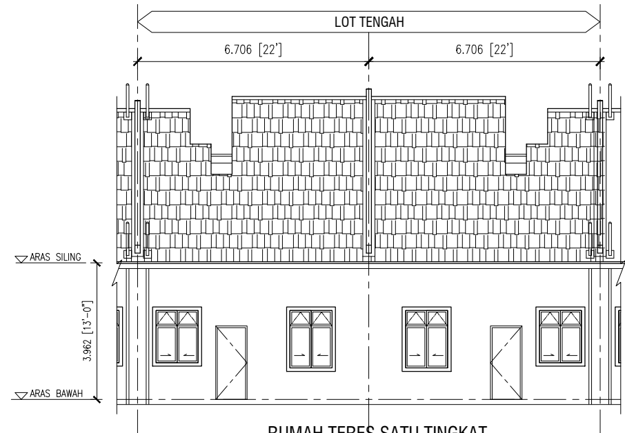
RUMAH TERES SATU TINGKAT PANDANGAN BELAKANG
