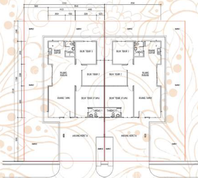
PELAN LANTAI
