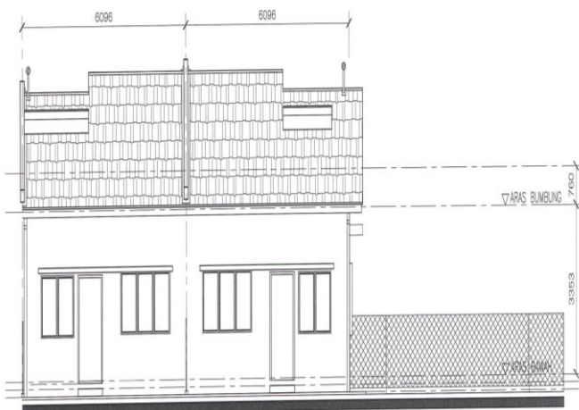
PANDANGAN BELAKANG
