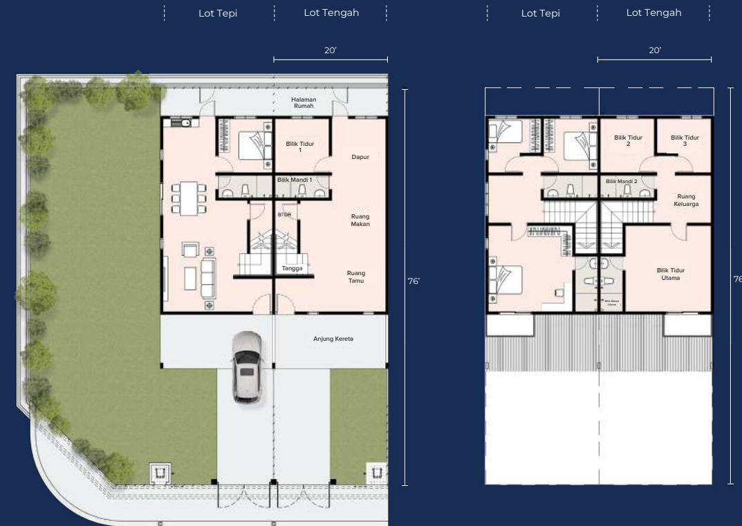
Pelan Tingkat Bawah
