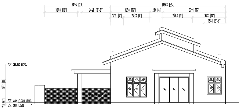
PANDANGAN KANAN RUMAH TERES 1 TINGKAT
