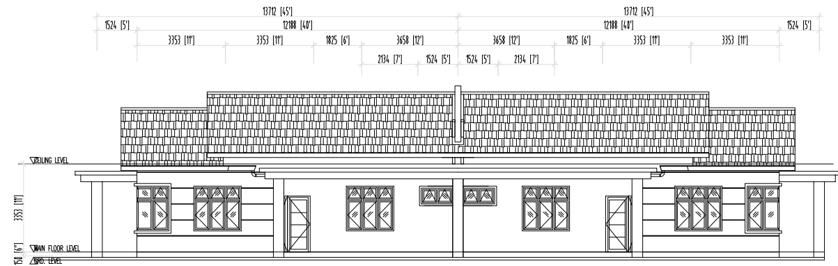
PANDANGAN HADAPAN RUMAH BERKEMBAR 1 TINGKAT
