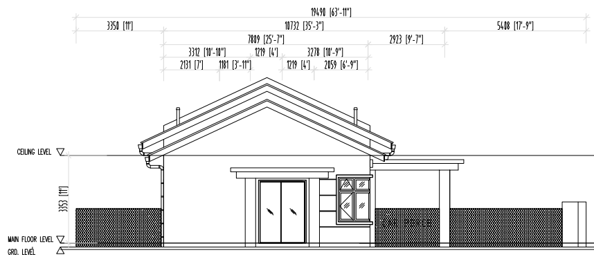
PANDANGAN KIRI RUMAH BERKEMBAR 1 TINGKAT
