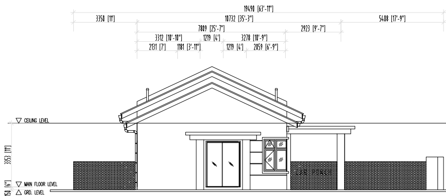
PANDANGAN KIRI RUMAH BERKEMBAR 1 TINGKAT
