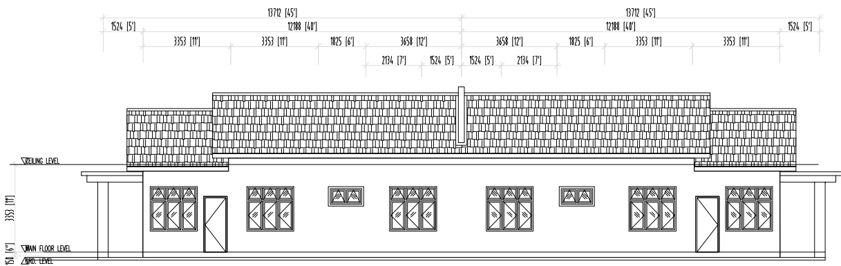
PANDANGAN BELAKANG RUMAH BERKEMBAR 1 TINGKAT
