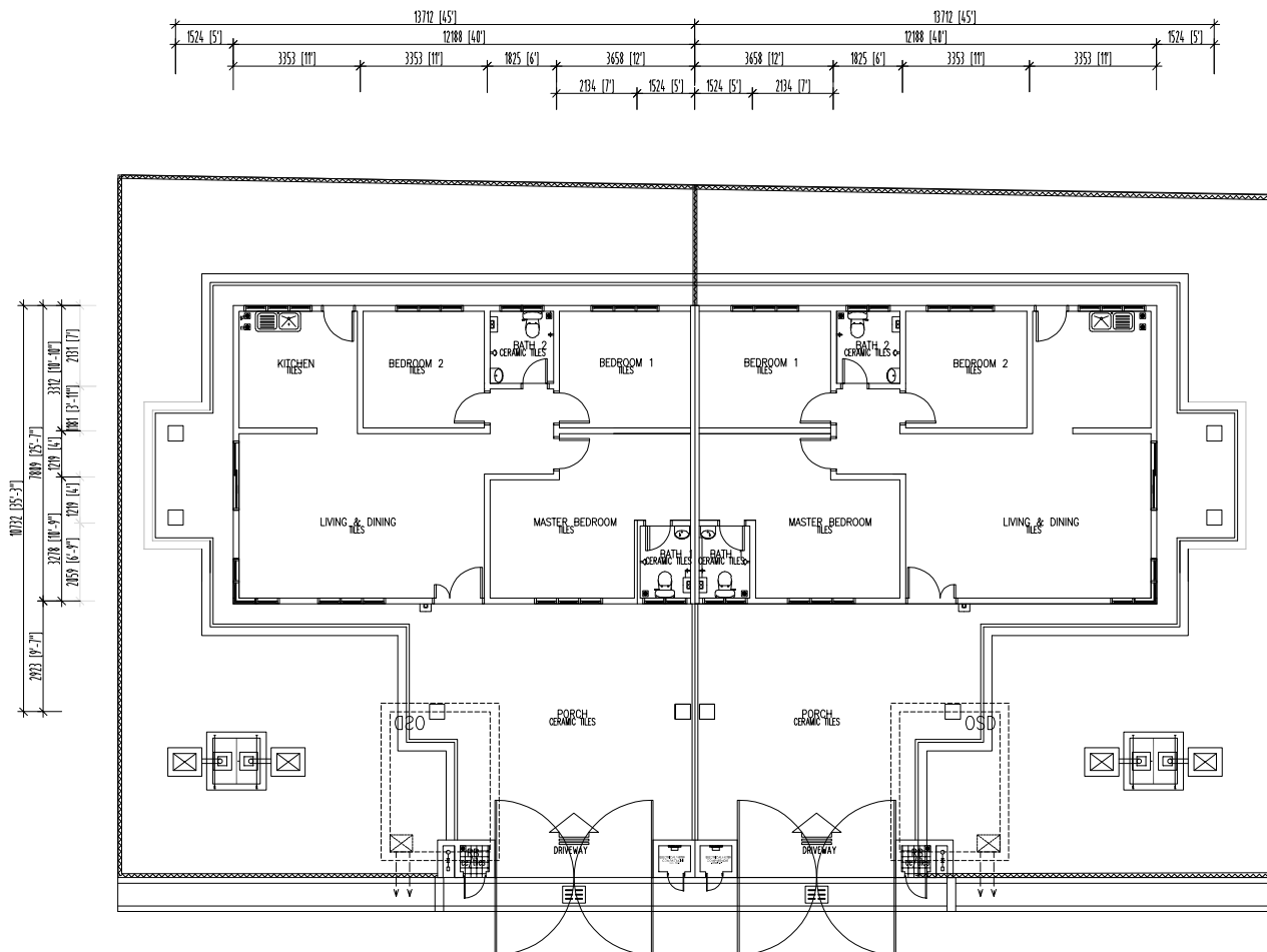
PELAN LANTAI TIPIKAL RUMAH BERKEMBAR 1 TINGKAT PELAN LANTAI ARAS TANAH
