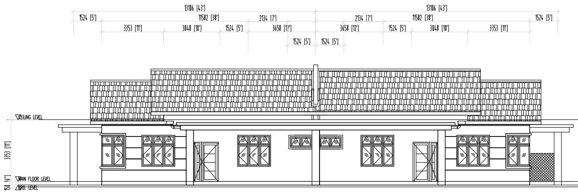
PANDANGAN HADAPAN RUMAH BERKEMBAR 1 TINGKAT
