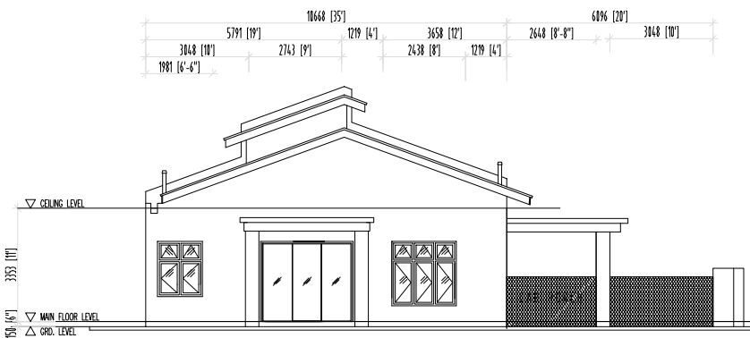
PANDANGAN KIRI RUMAH TERES 1 TINGKAT
