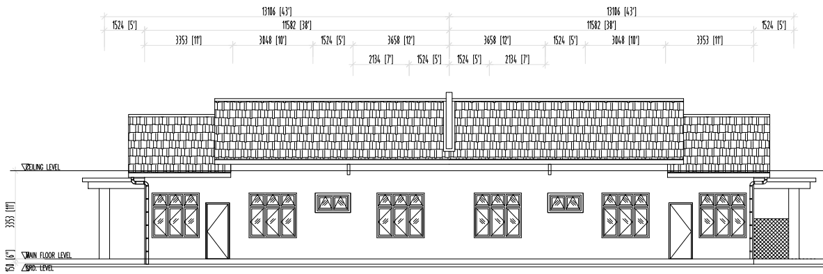
PANDANGAN BELAKANG RUMAH BERKEMBAR 1 TINGKAT
