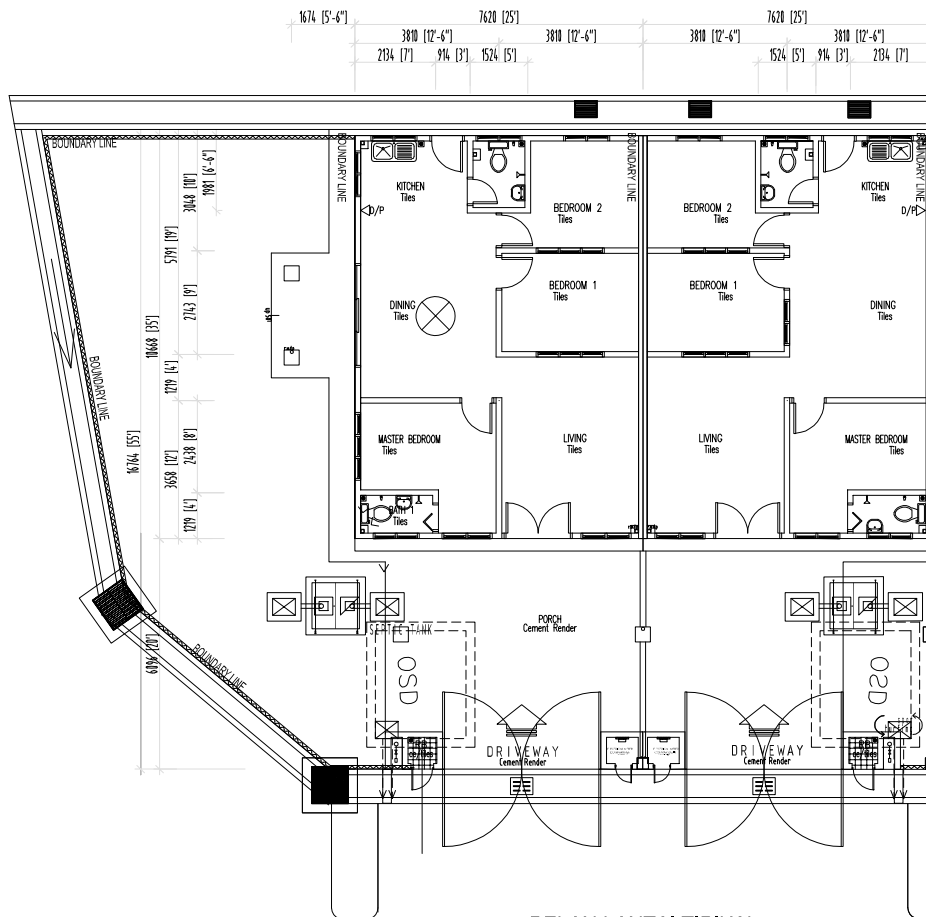
PELAN LANTAI TIPIKAL RUMAH TERES 1 TINGKAT PELAN LANTAI ARAS TANAH
