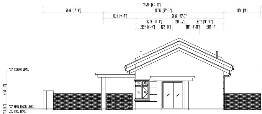
PANDANGAN KANAN RUMAH BERKEMBAR 1 TINGKAT
