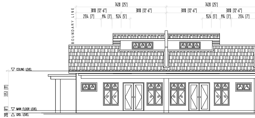
PANDANGAN HADAPAN RUMAH TERES 1 TINGKAT
