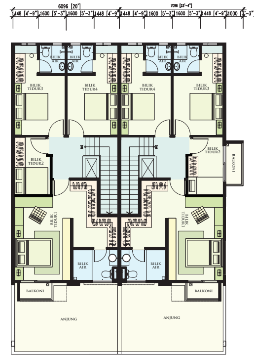
PELAN LANTAI &amp; SPESIFIKASI BANGGUNAN
