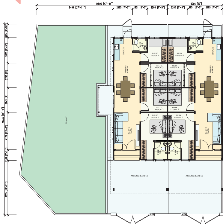
PELAN LANTAI &amp; SPESIFIKASI BANGGUNAN
