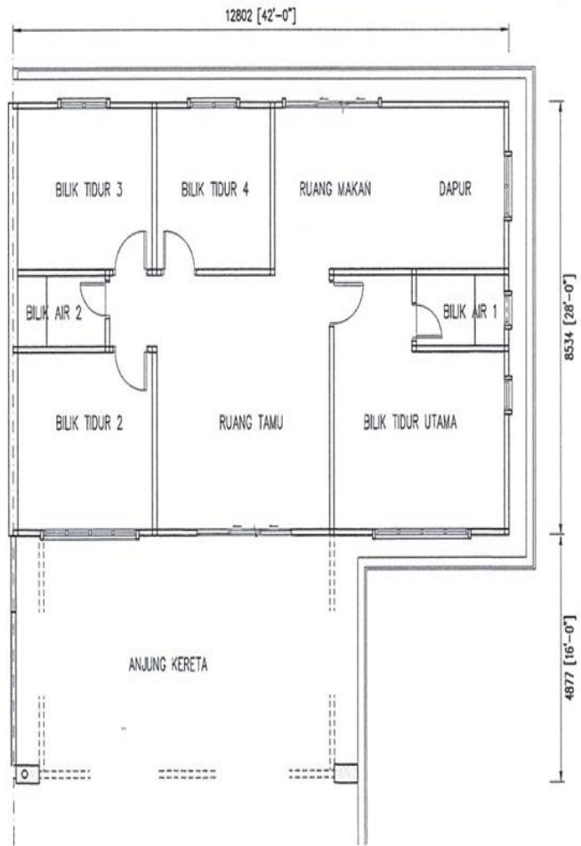
PELAN LANTAI
